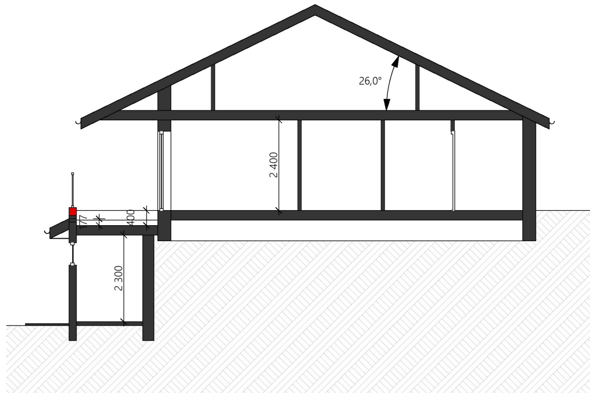
SNITT C-C
