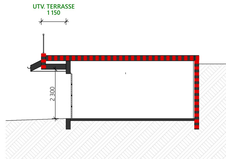
SNITT D-D
