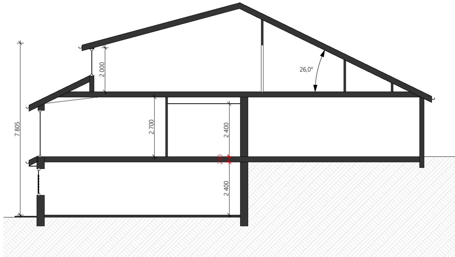
SNITT A-A
