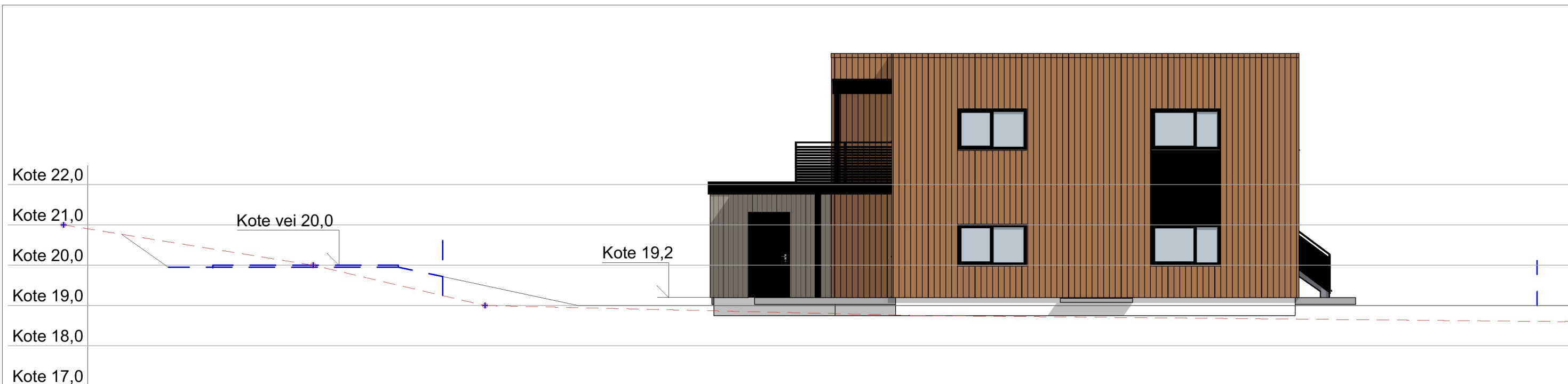
1:100 Fasade Øst
