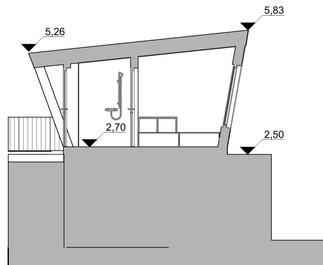
1:100 Snitt D-D
