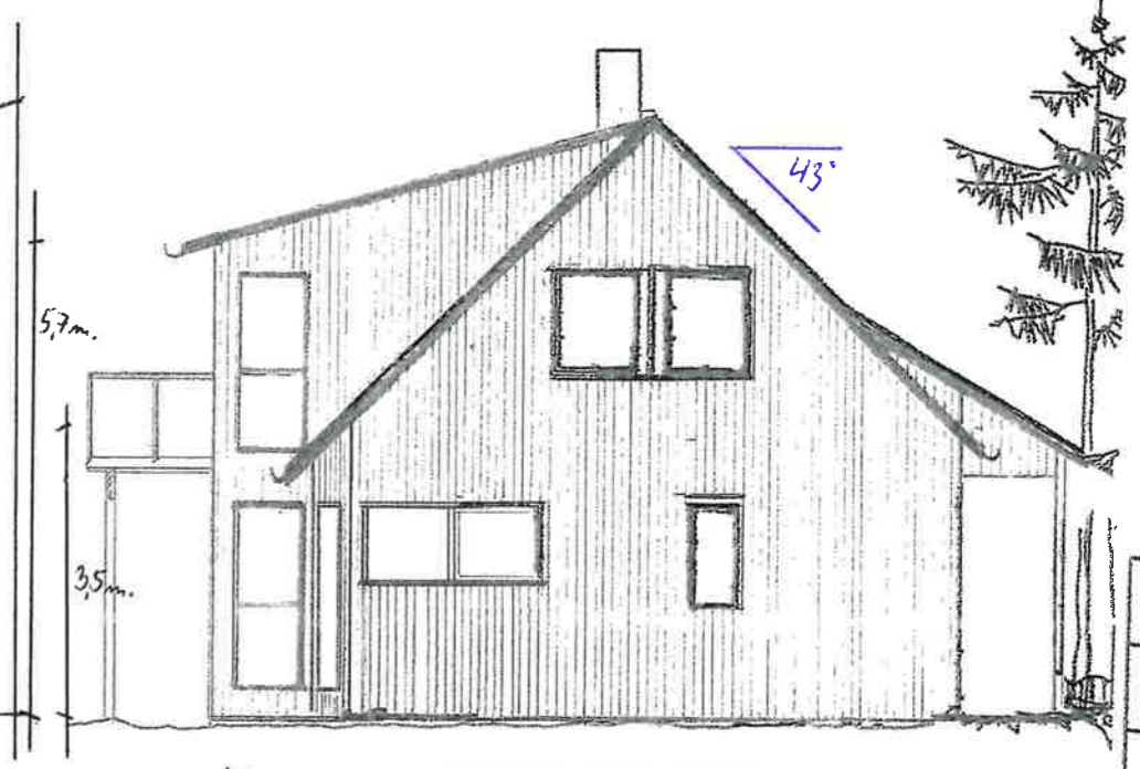
FASADE MOT NORD, NY
