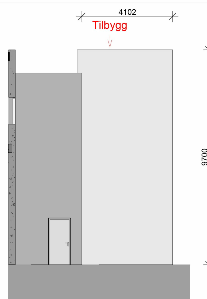
Fasade ØST Byggetrinn 3 1 : 100
