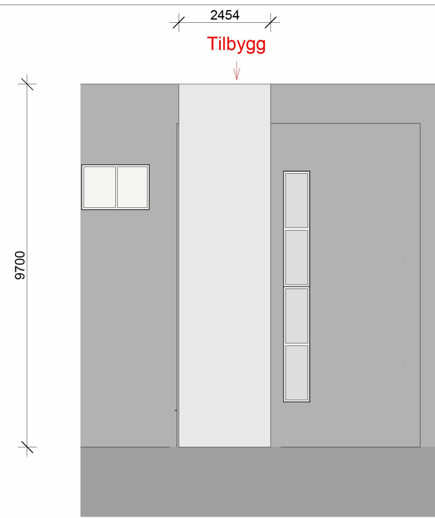
Fasade NORD Byggetrinn 3 1 : 100
