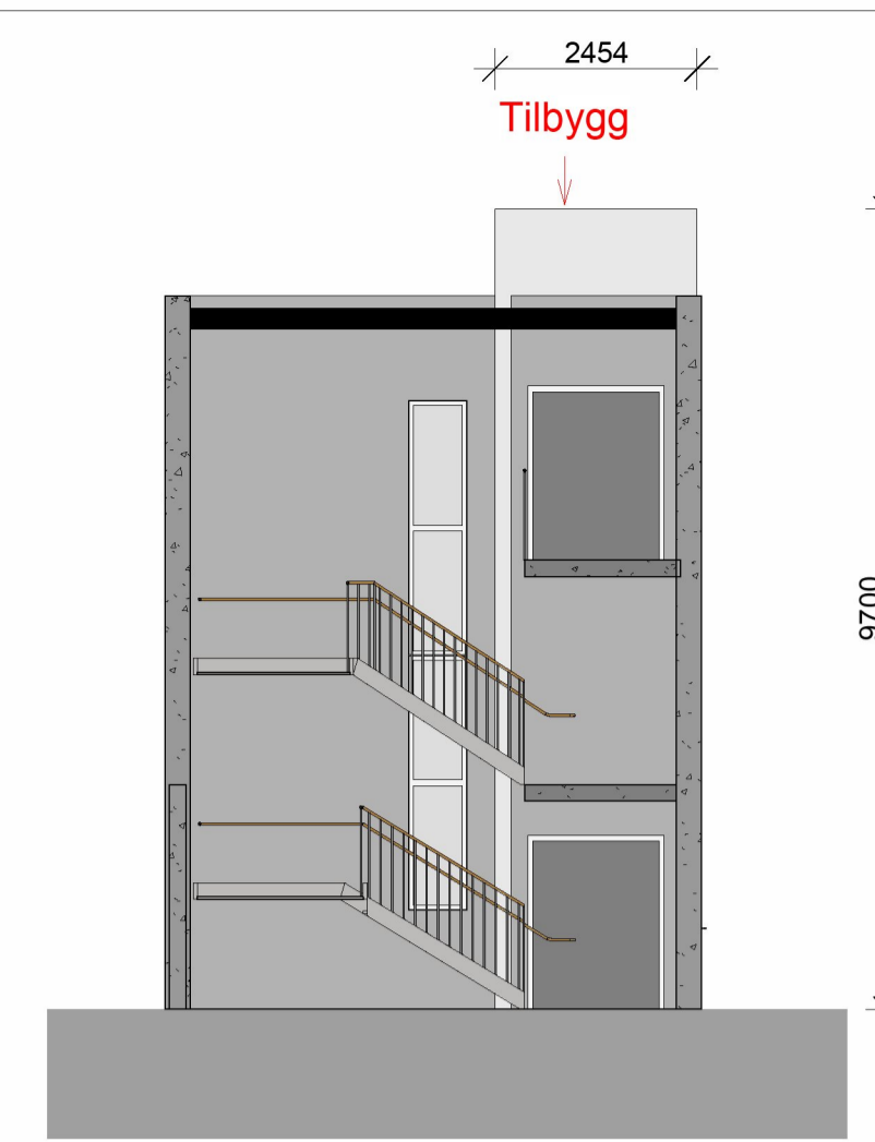
Oppriss gjennom trapperom SØR 1 : 100
