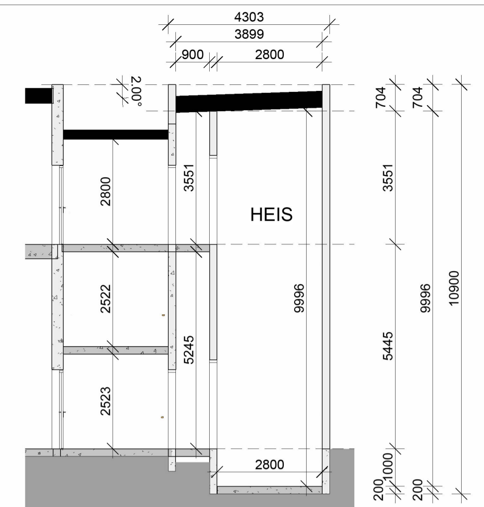
Snitt 5-5 1 : 100
