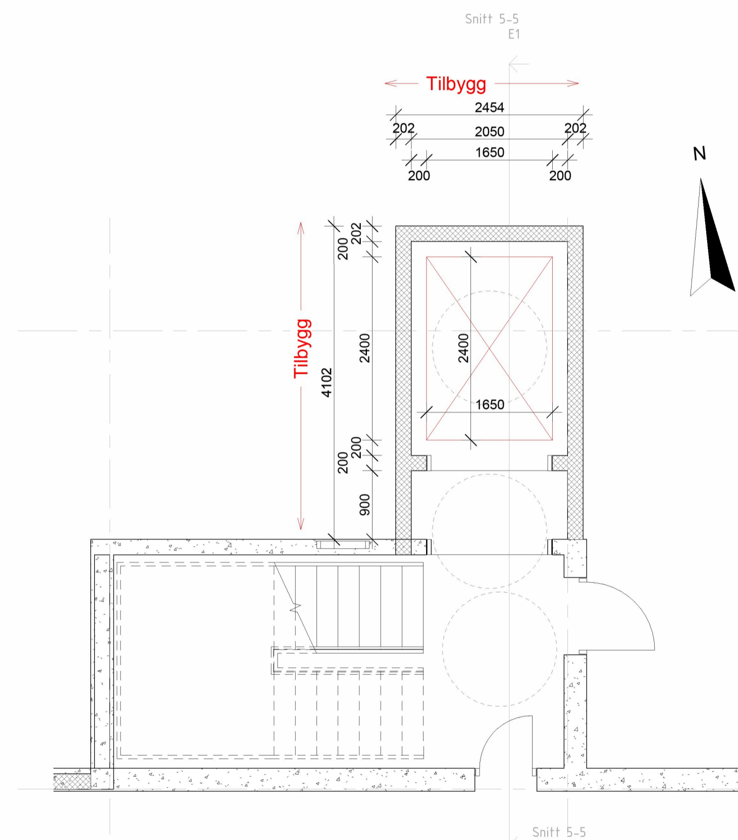
Plan 01 Byggetrinn 3 1 : 50
