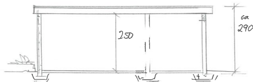
SNITT
