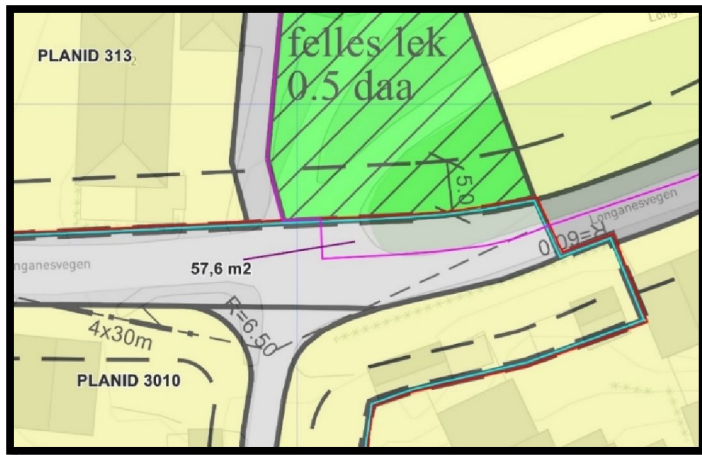
Figur 14 – Planforslag linje (rosa) over eksisterende detaljplan med plangrense i rød, viser overlapping av planer.
