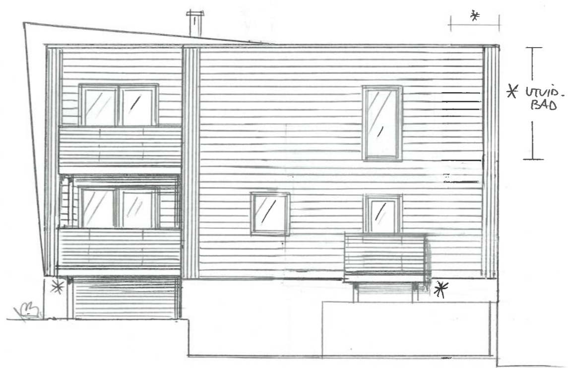
FASADE SØR
