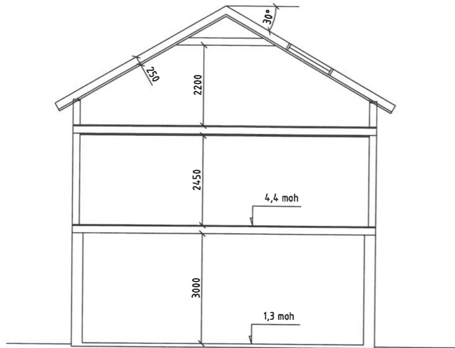
Snitt A-A
