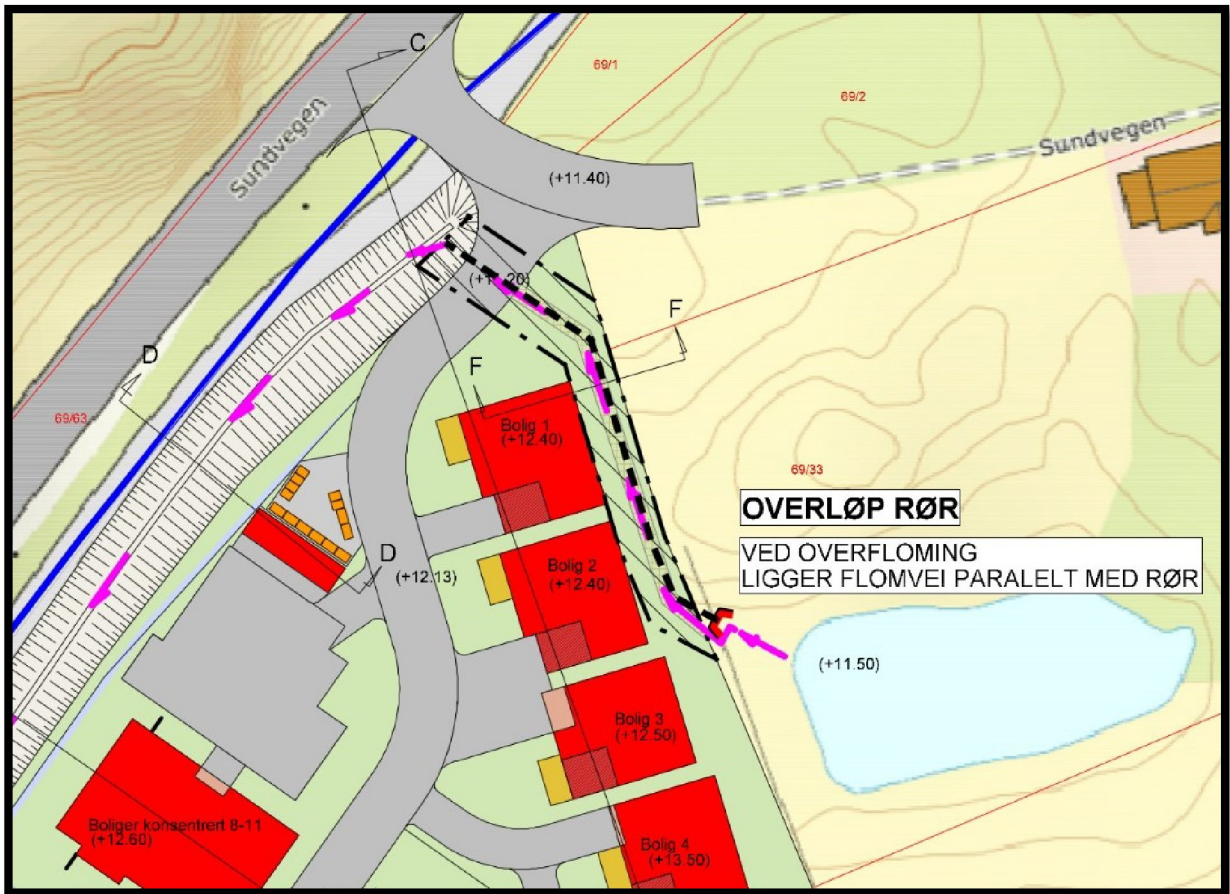
Figur 17. – Skisse løsning, to alt.
