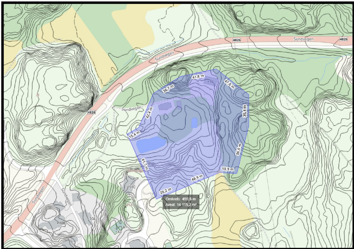
Figur 15. – Nedslagsfelt
