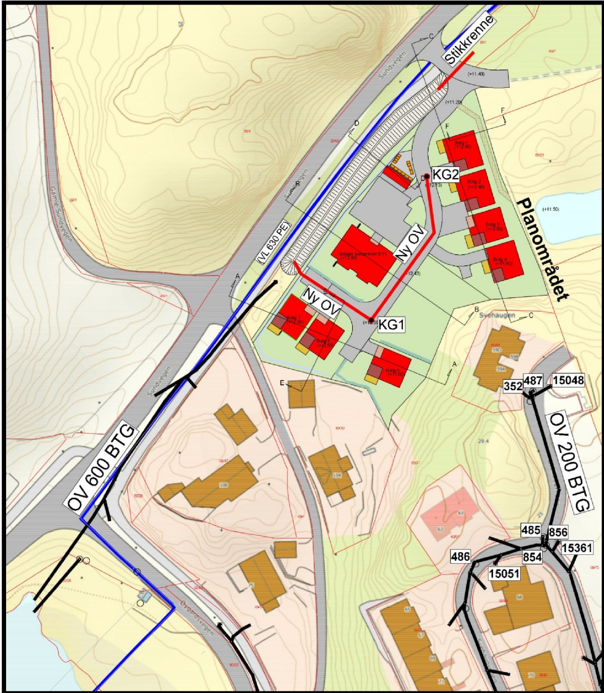
Figur 10. – Overvannsledning.
