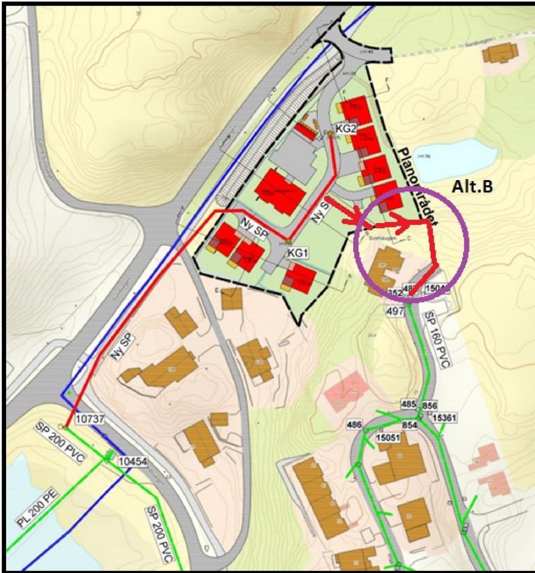
Figur 09. – Spillvannsledning.
