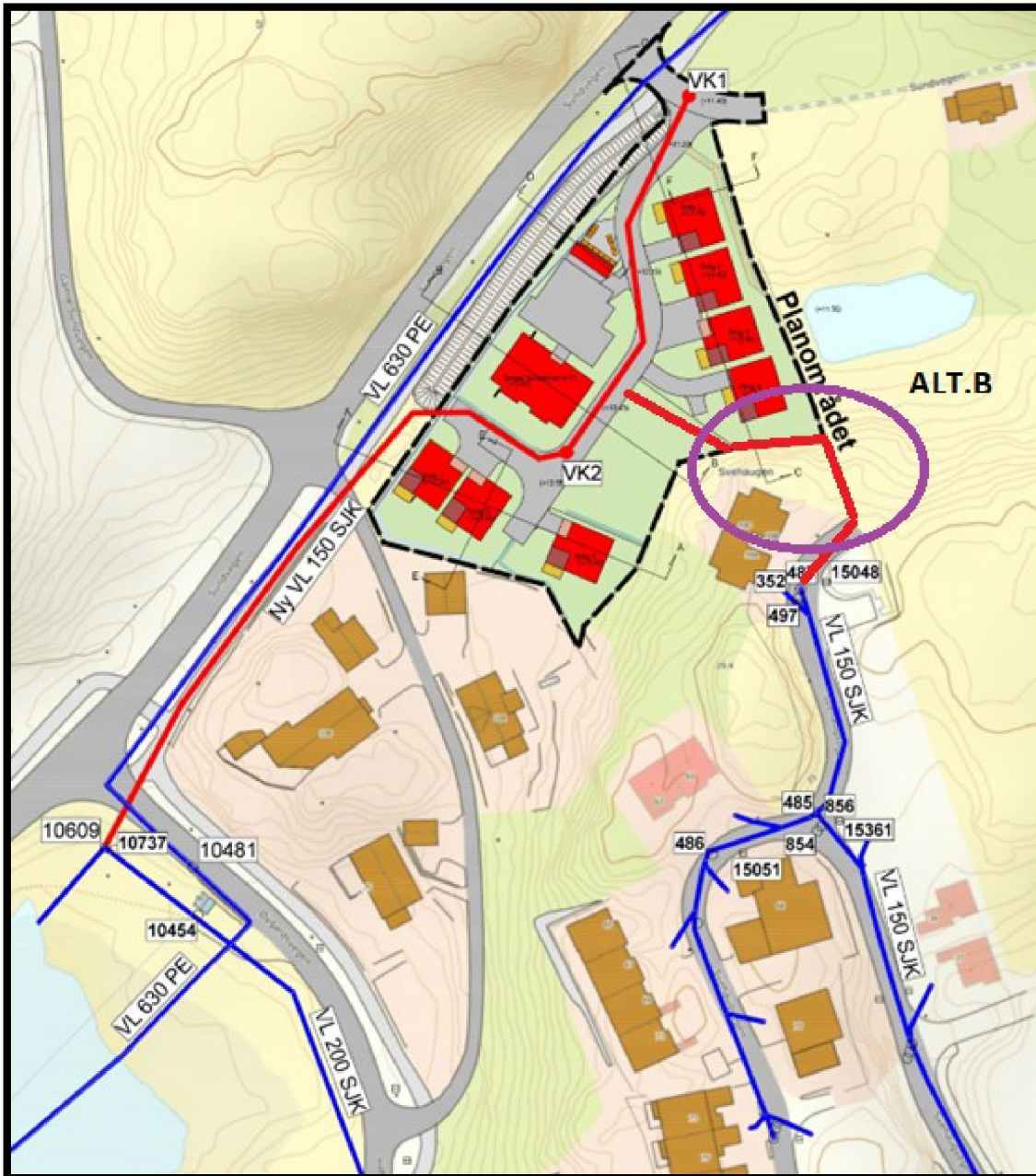
Figur 07. – Vannledning.
