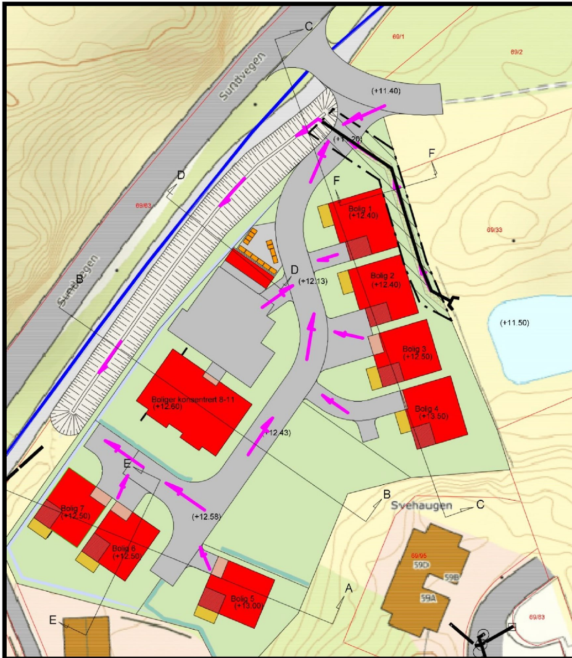
Figur 11. – Flomvei.
