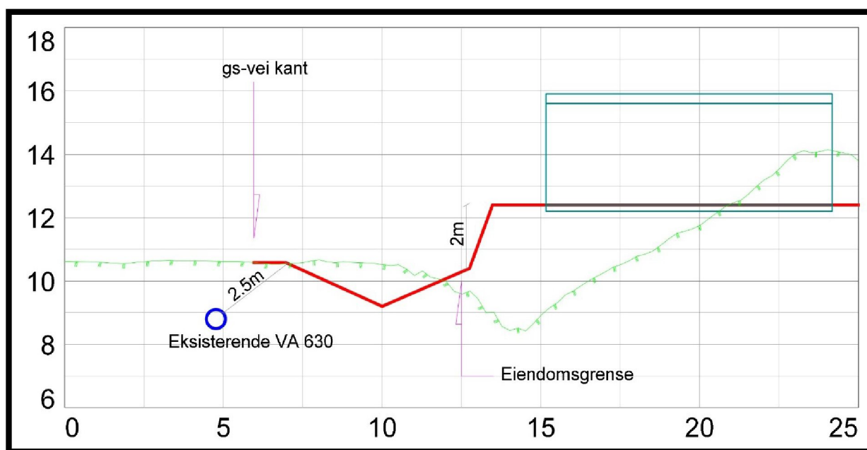
Figur 12. – Snitt D - Justering grøft.
