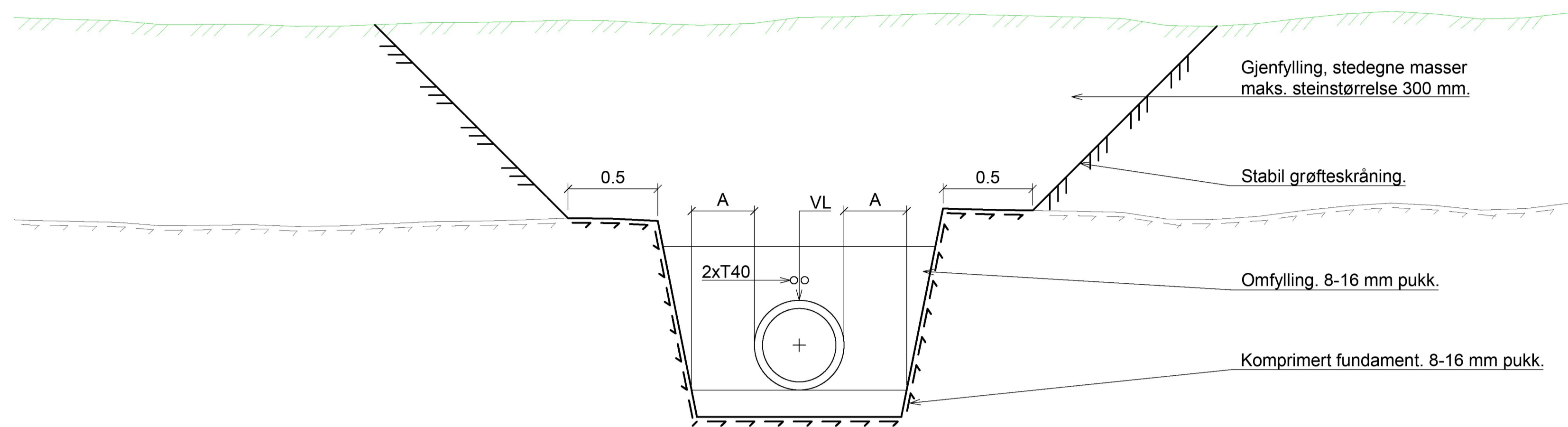
Grøftesnitt
