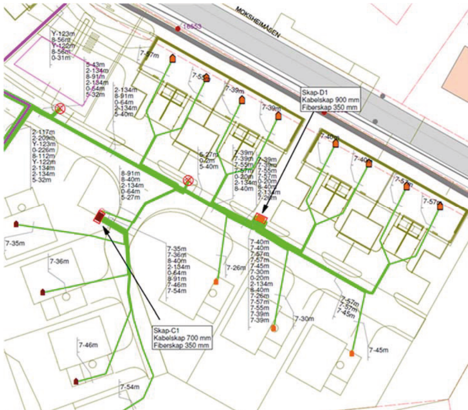
Figur 23 Eksempel på kabelplan med snittmerking
