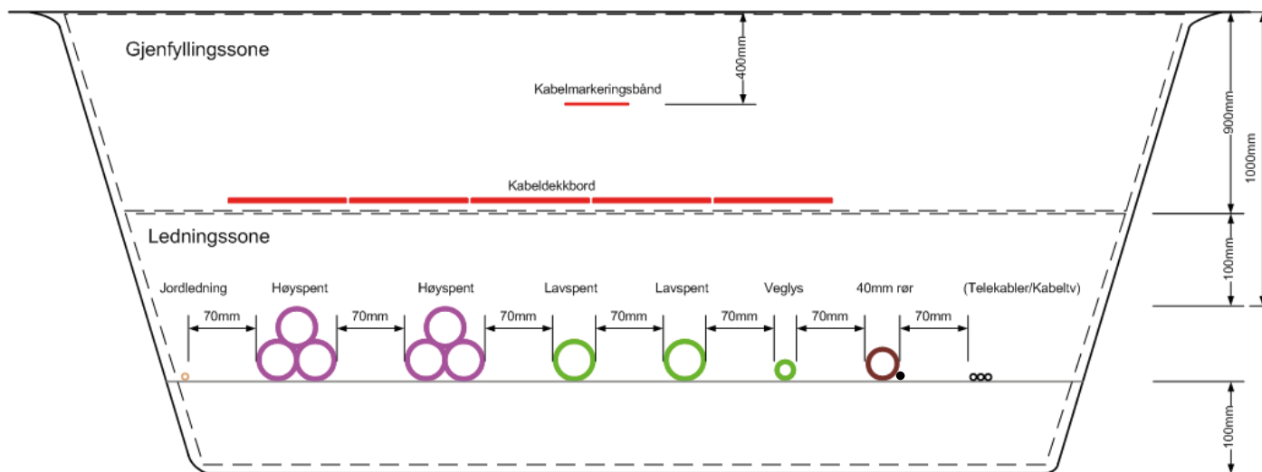
Figur 2. Grøftesnitt i dyrket mark.
