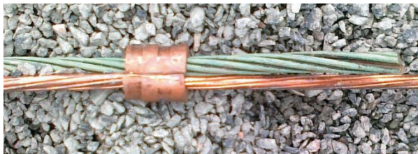
Figur 29. Skjøting av jordledning med C-press
