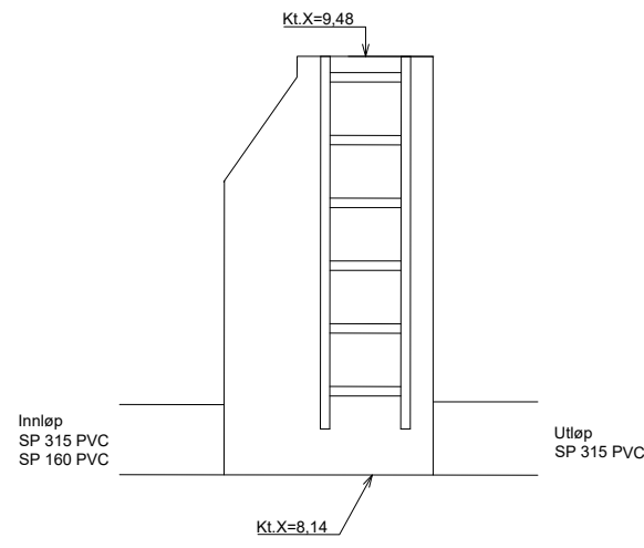
Rennekum SK2 Snitt A-A
