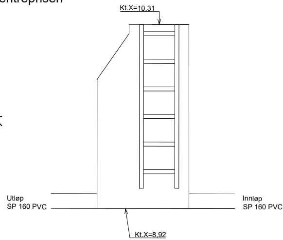
Rennekum SK4 Snitt A-A
