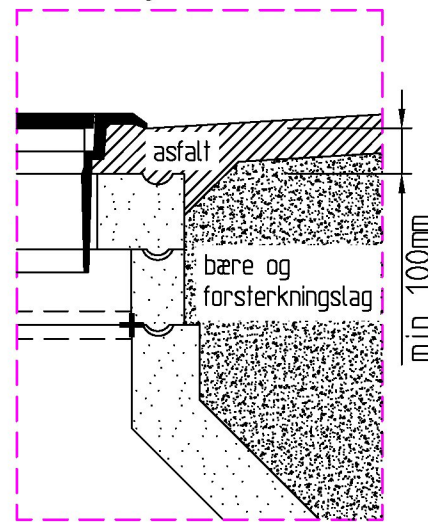
Detalj A 1:10
