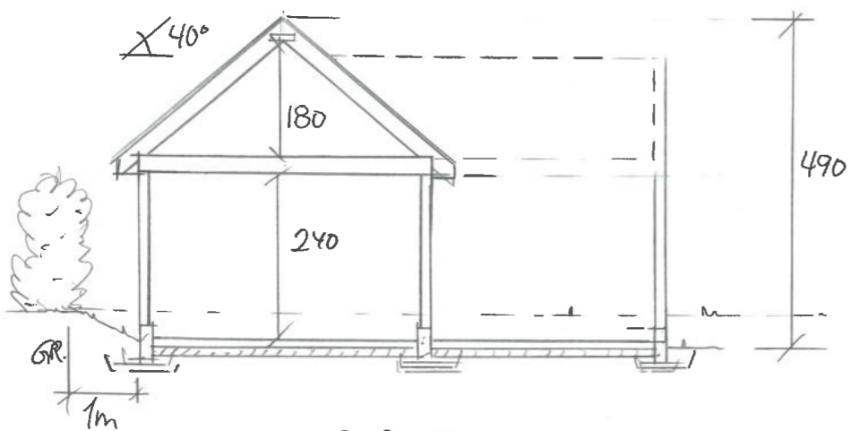
SNITT
