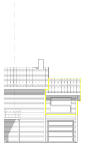
1:100 Fasade Nord
