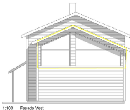
1:100 Fasade Vest
