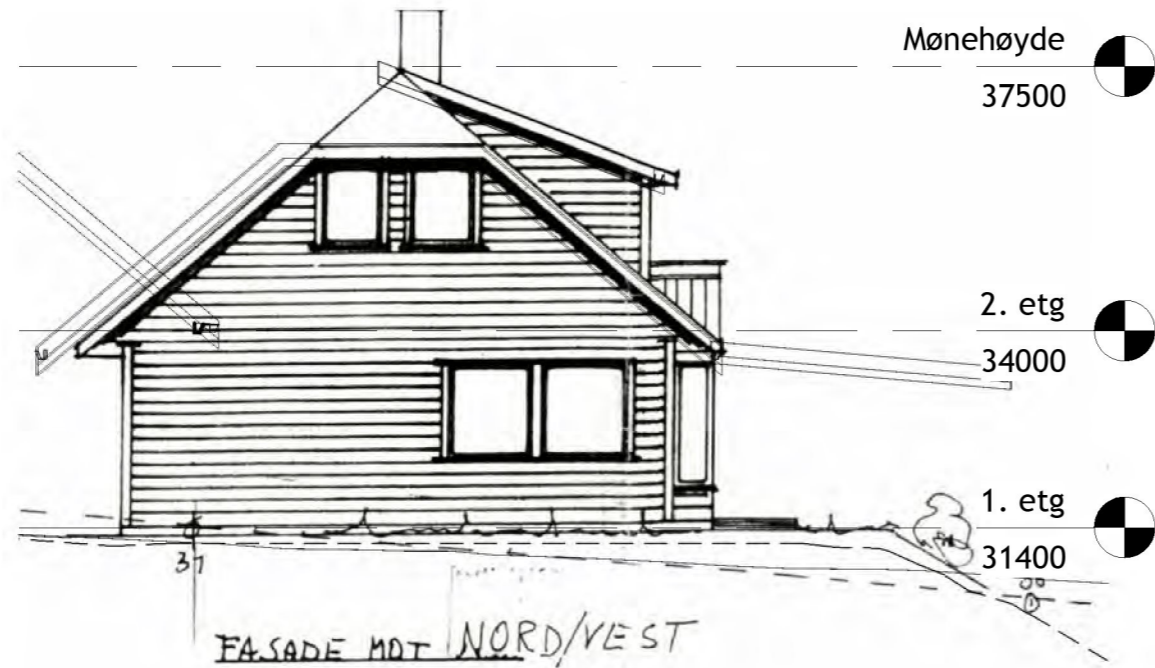
1 Eksis. fasade nordvest 1 : 100
