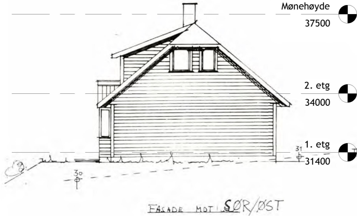
3 Eksis. fasade sørøst 1 : 100
