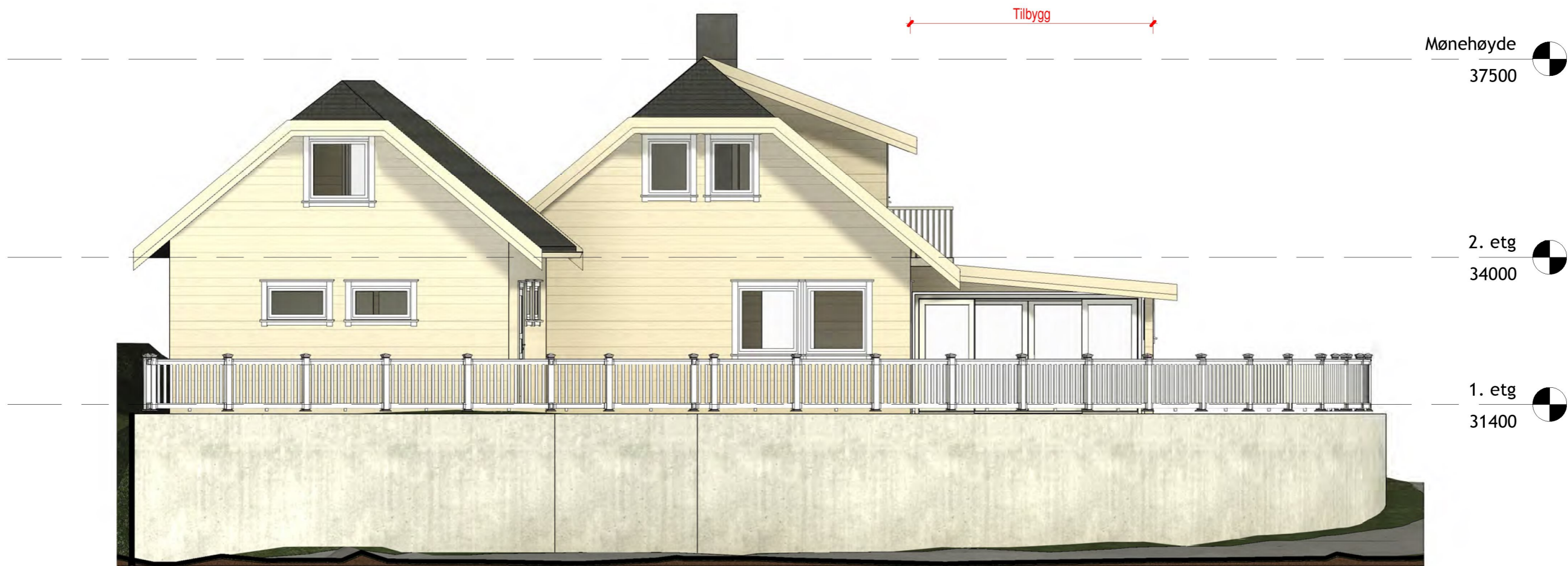
5 Fasade nordvest 1 : 75
