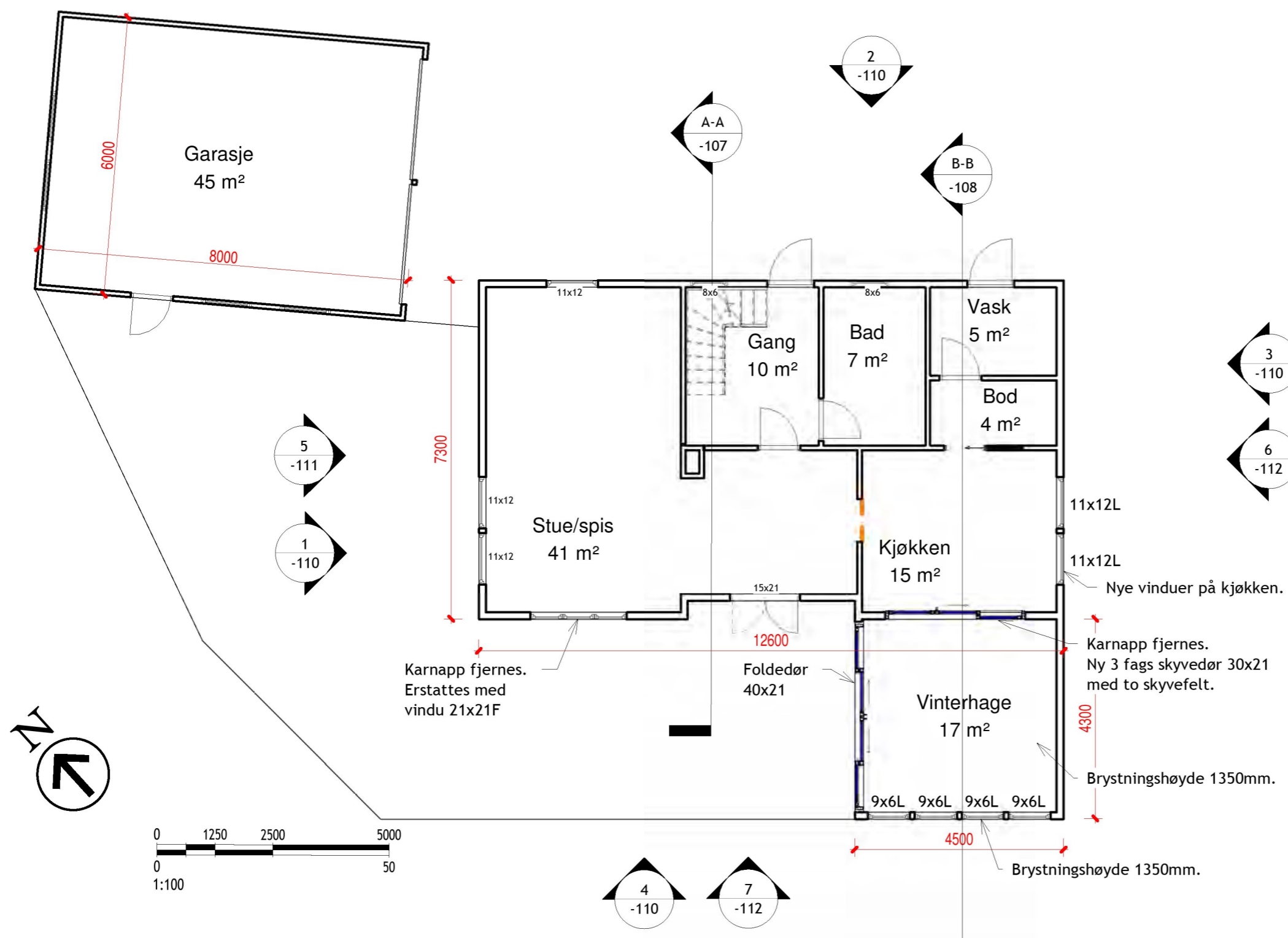
1 Plan 1. etasje 1 : 100
