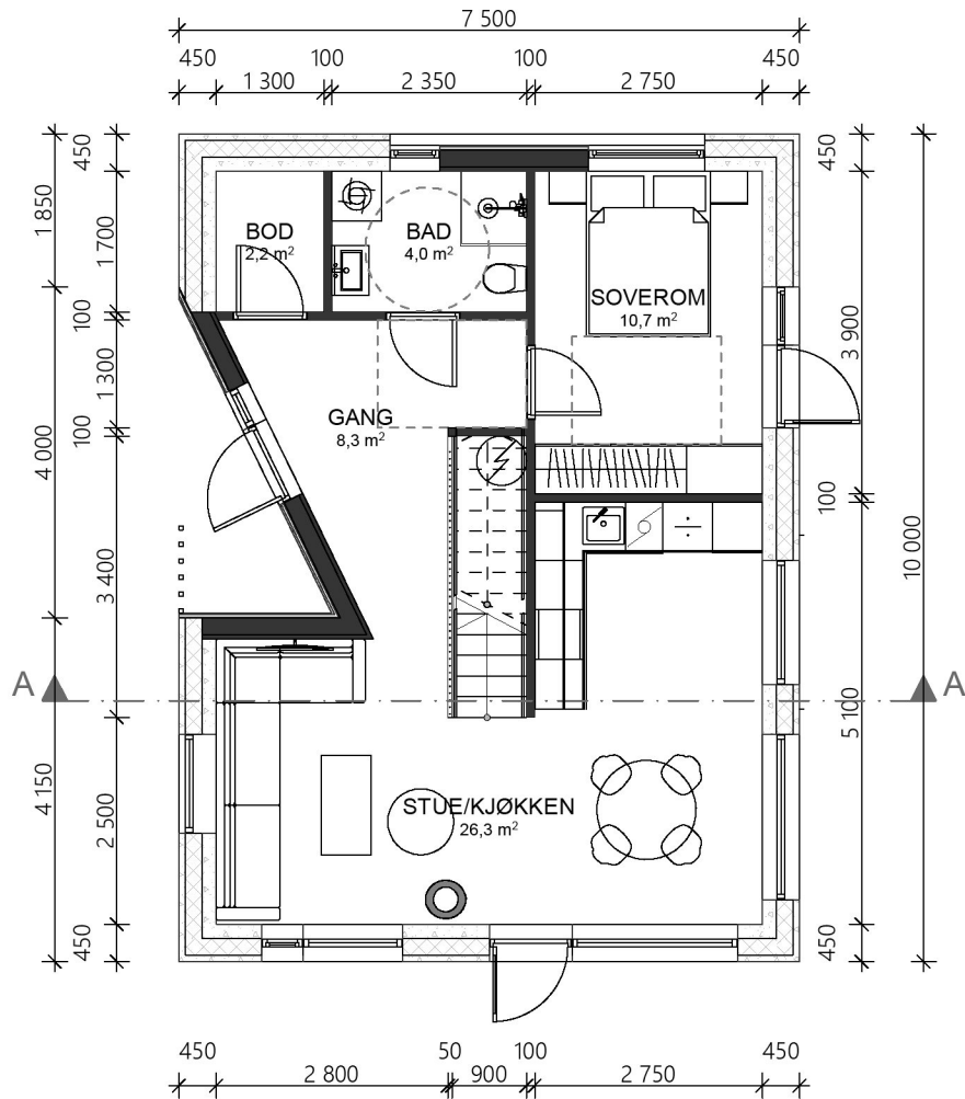
PLAN HOVEDETASJE
