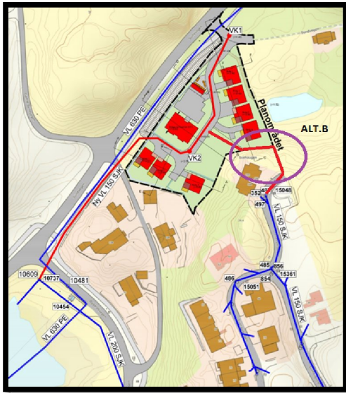
Figur 59 – Vannledning.
