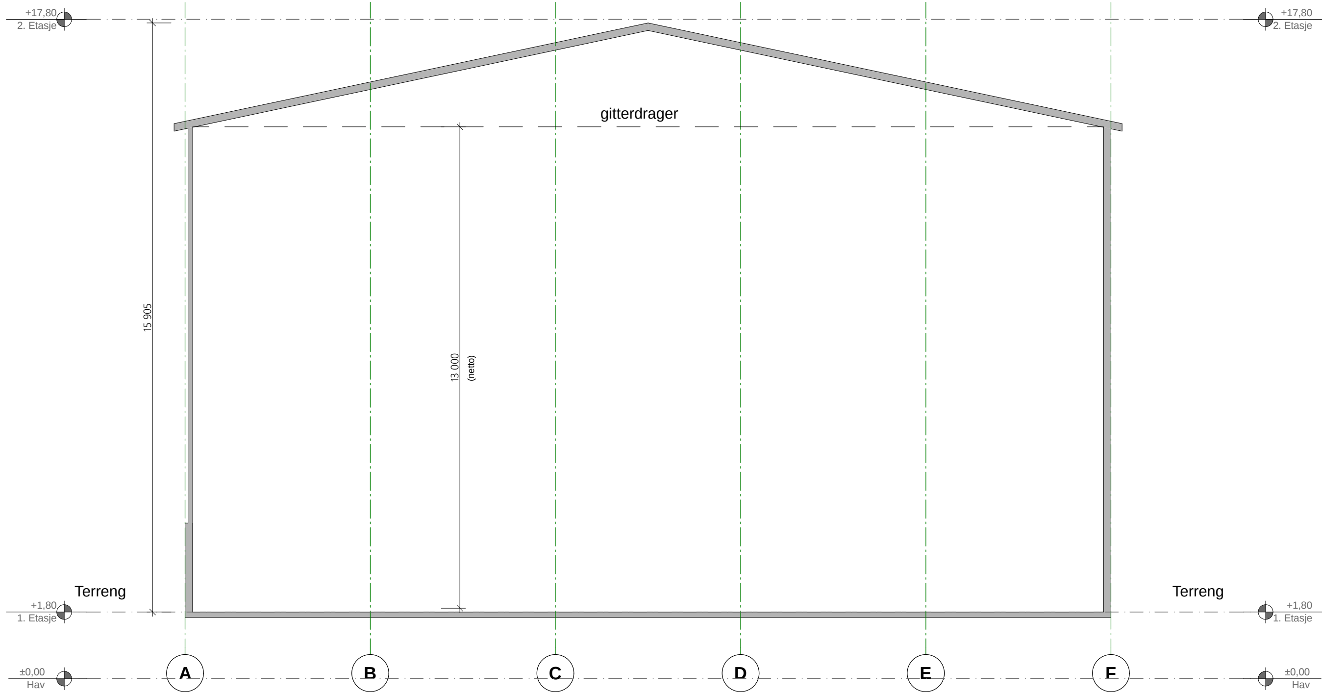
1:100 Snitt A
