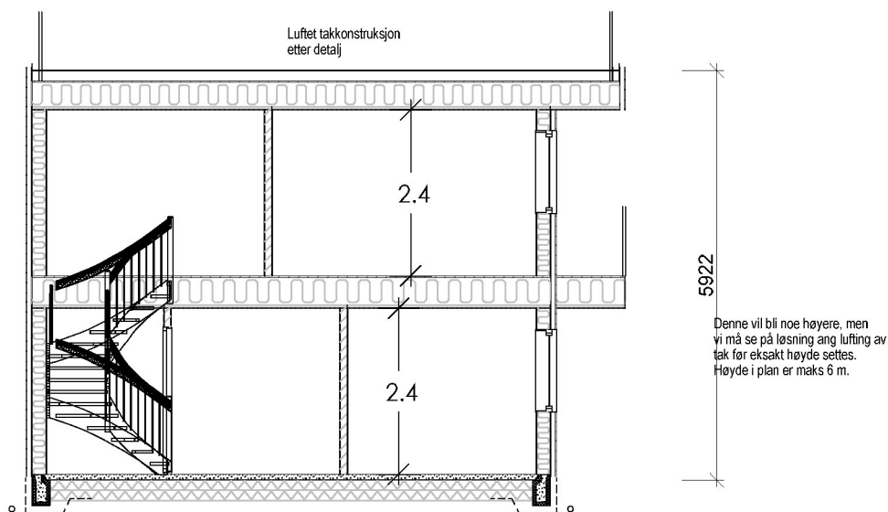
Snitt A:A
