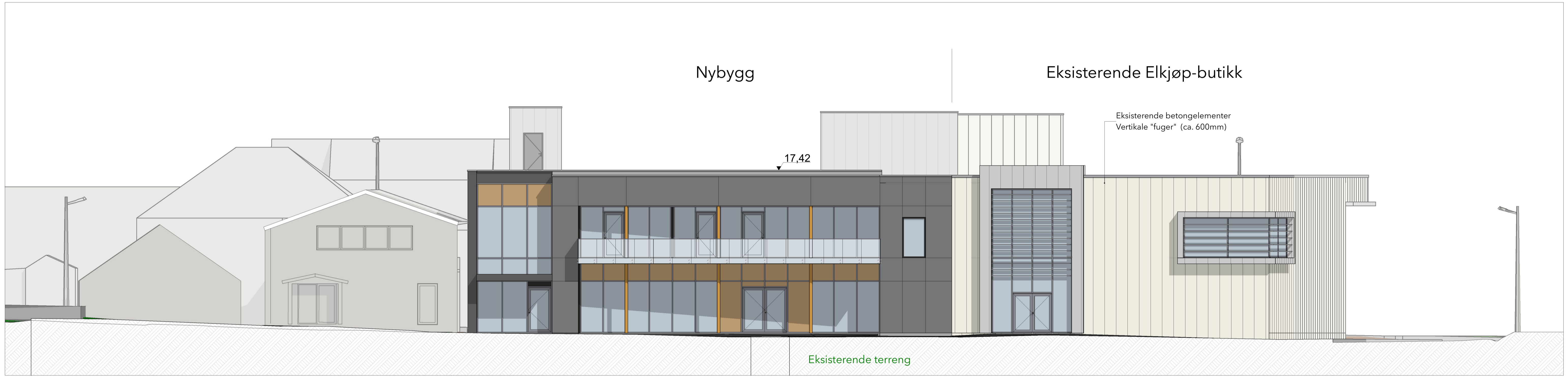
1:100 Fasade Vest
