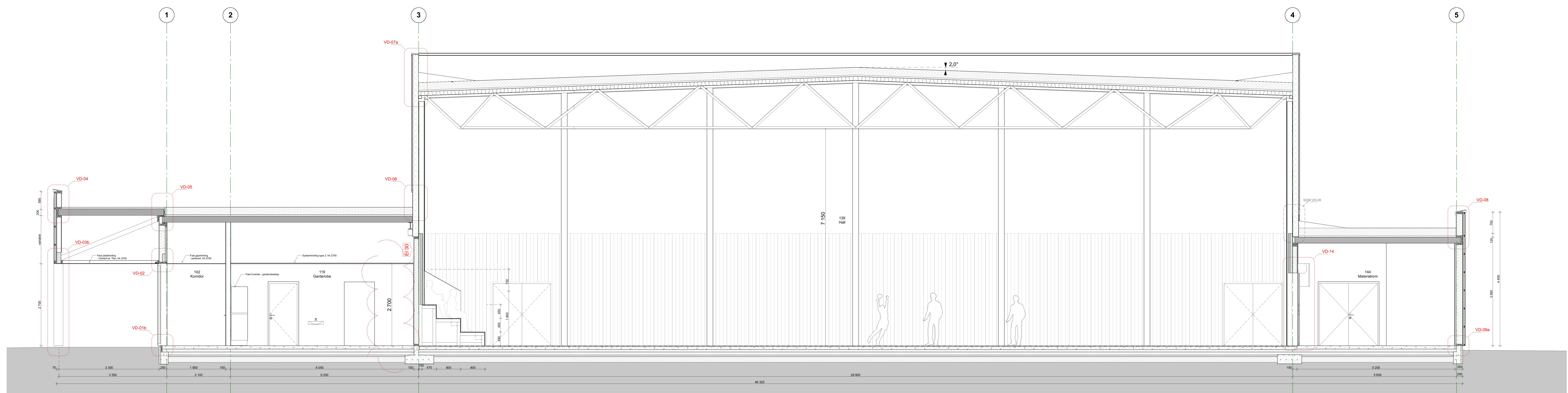
Snitt B-B
