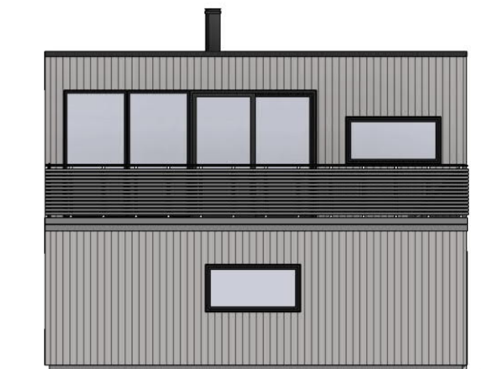
Sør 1 : 100
