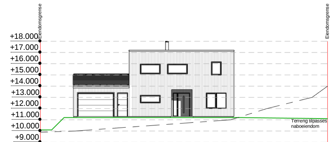
Terrengsnitt Øst 1 : 200
