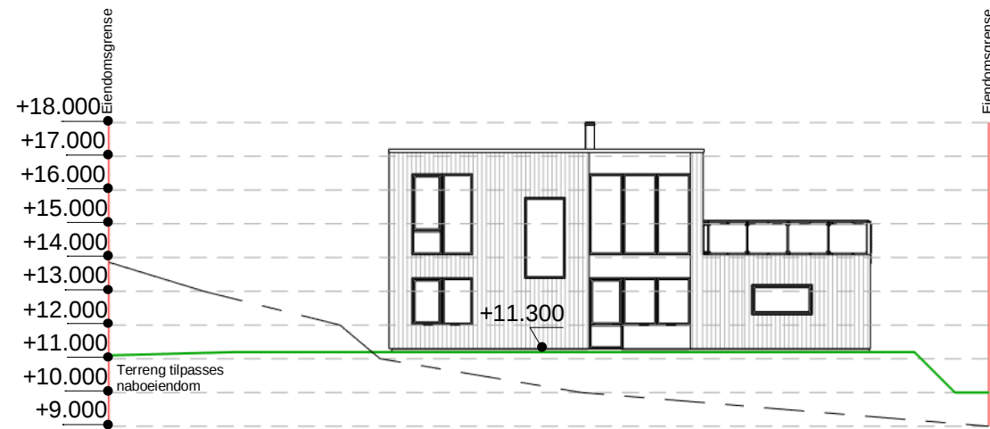
Terrengsnitt Vest 1 : 200
