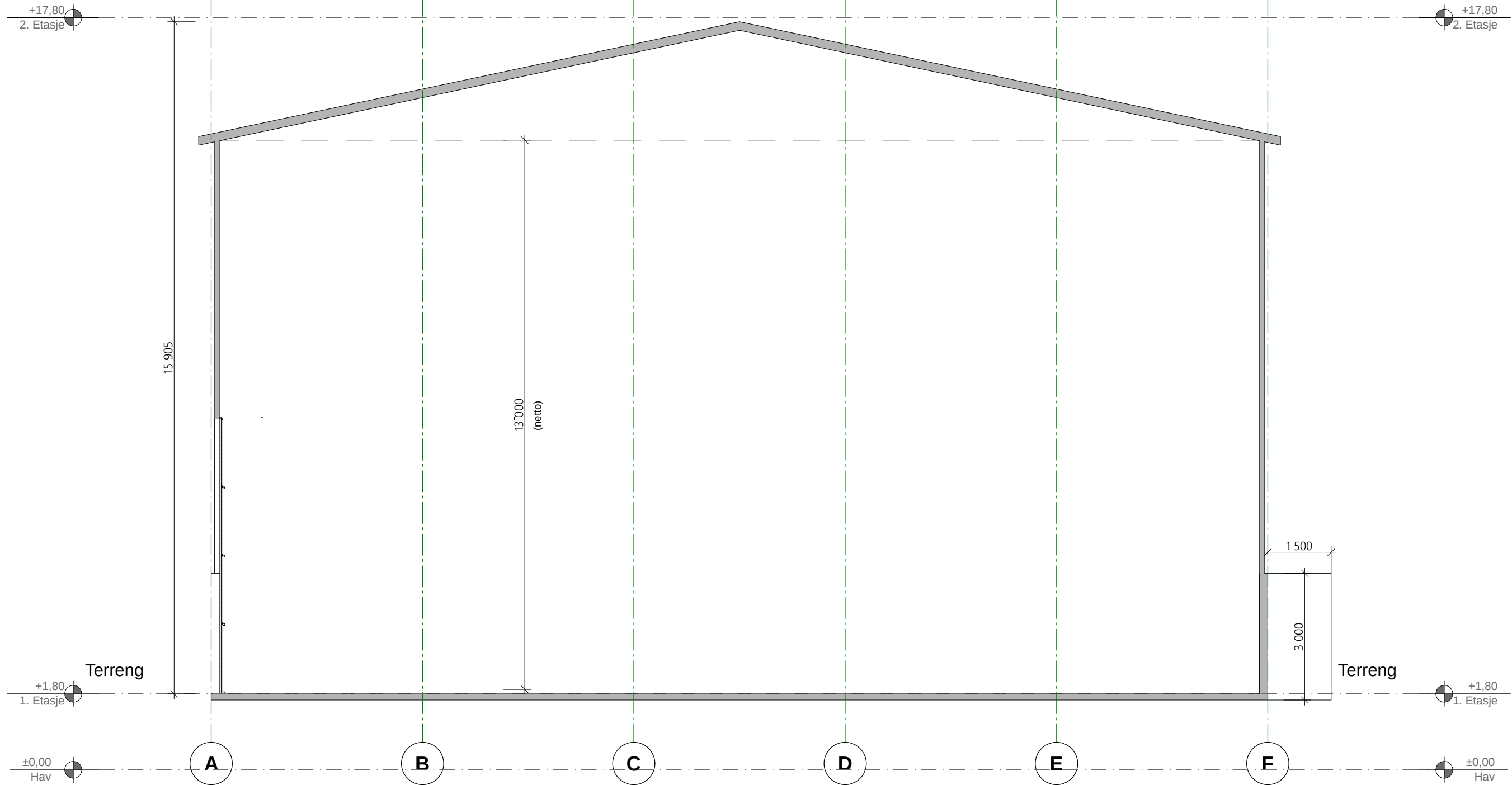
1:100 Snitt A
