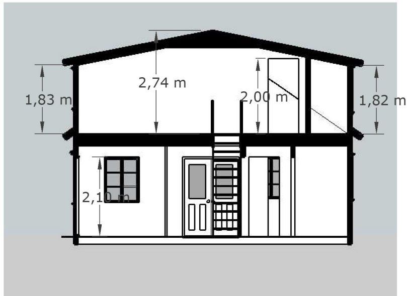
Snitt Vest
