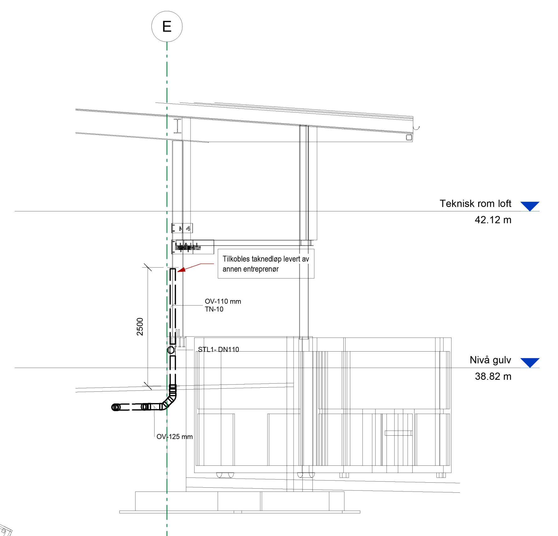
2 Prinsipp taknedløp 1 : 50
