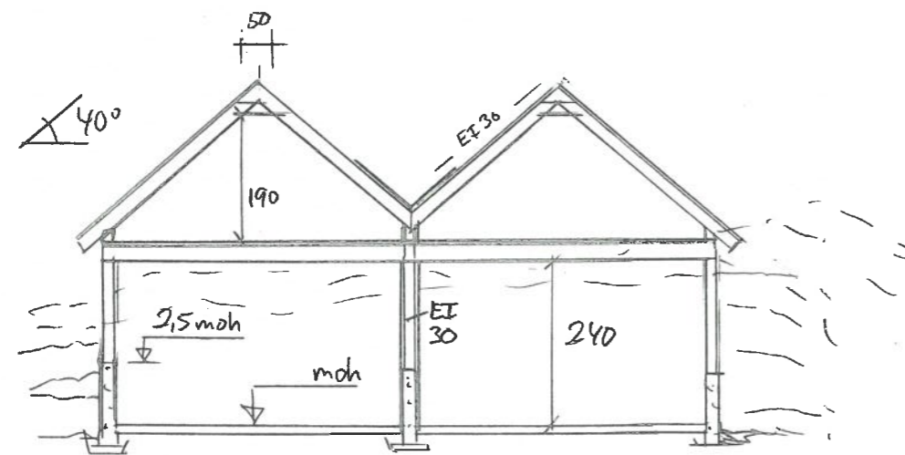
SNITT
