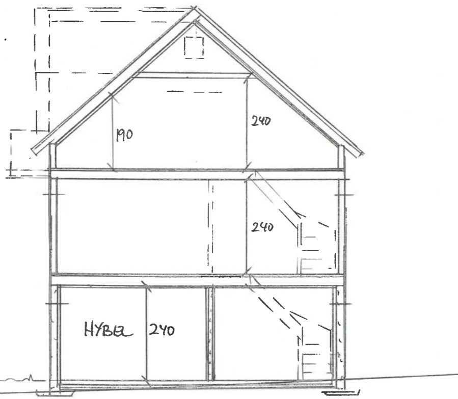
SNITT
