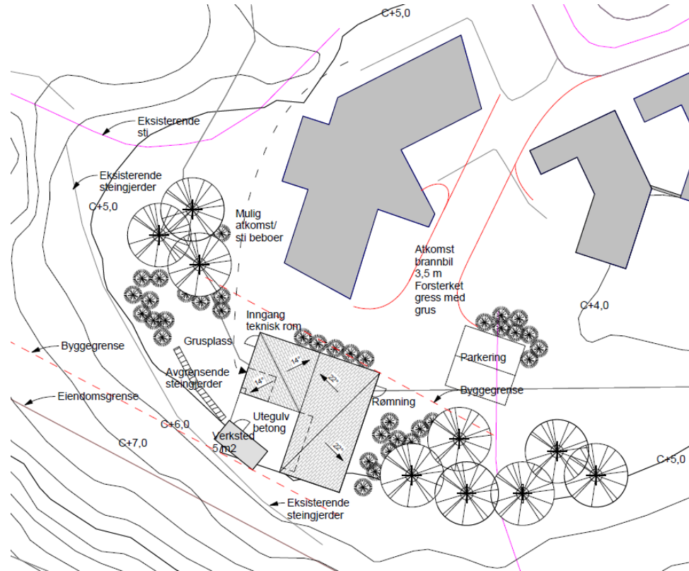
Figur 1: Utomhusplan
