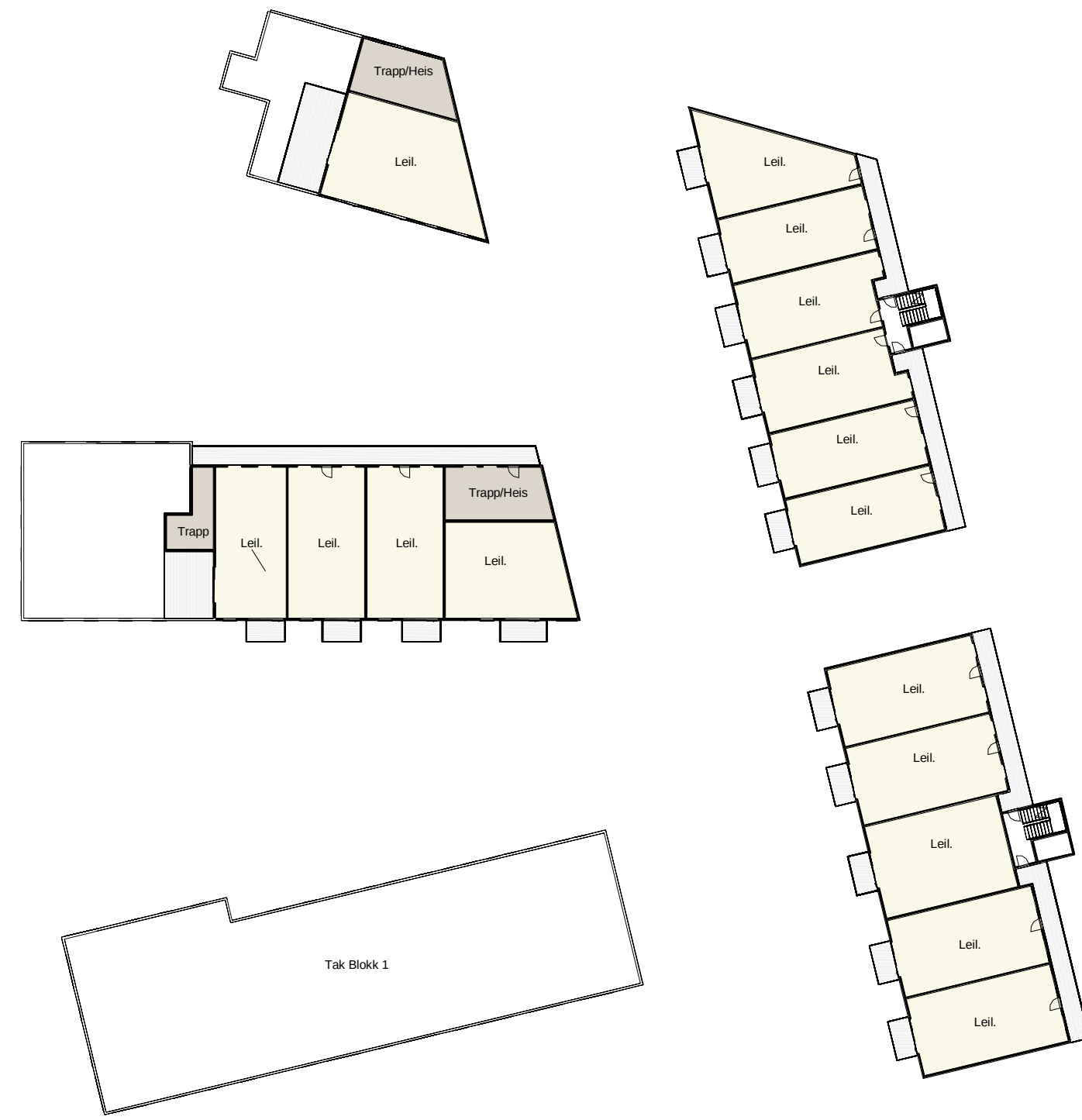
Et. 6 nederste nivå / Et. 2 Øverste nivå
