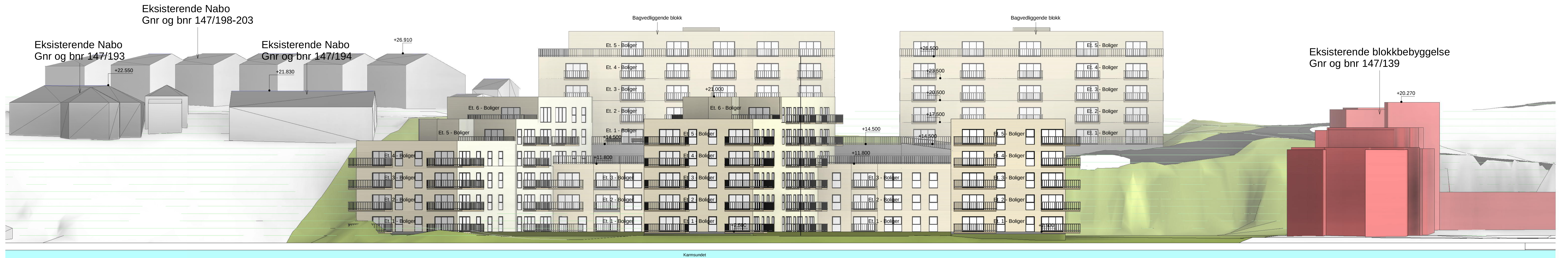
Terrenngnitt 1-1 1 : 200
