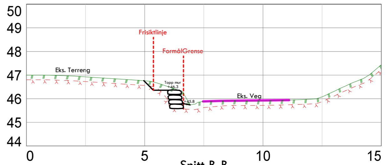
Snitt A-A
