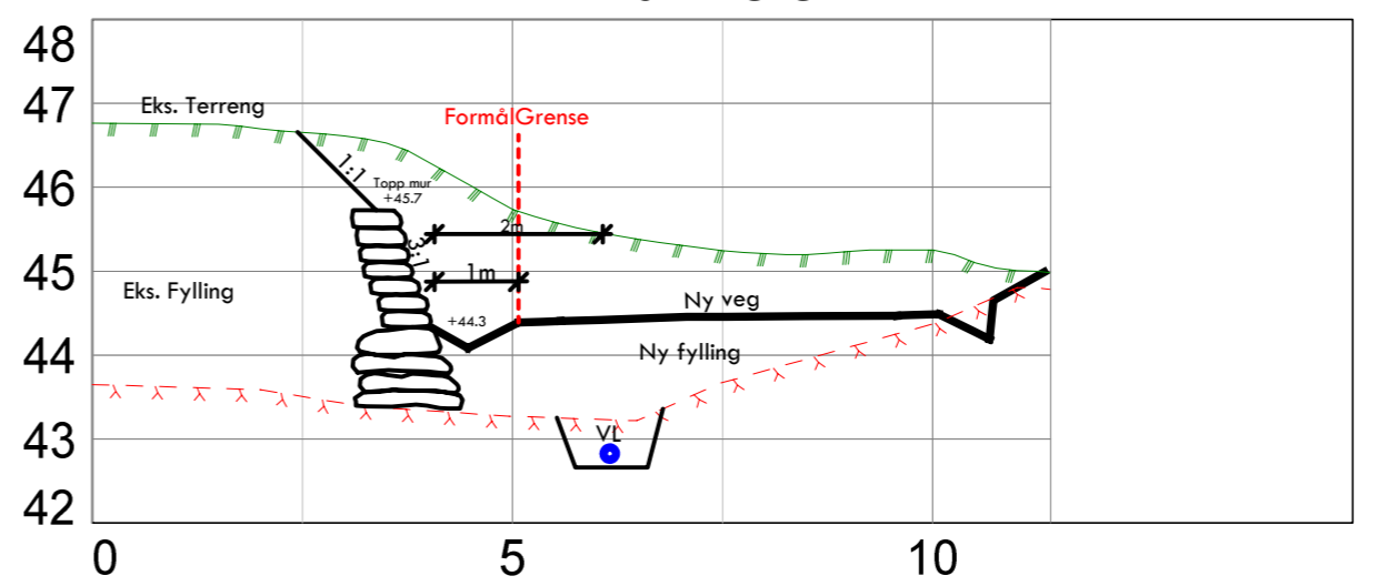
Snitt C-C
