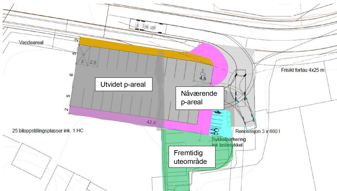
Figur 6 Skisse av parkeringsplass etter utvidelse. Areal lengst sør på dagens parkeringsplass vil bli opparbeidet til lekeareal i tråd med utomhusplan som er under utarbeidelse. Rosa skravur er gangareal, oransje skravur er areal mellom p-plass og fortau langs Tostemvegen (kilde: Norconsult)
