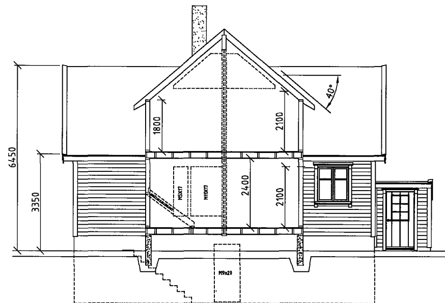
SNITT B-B
