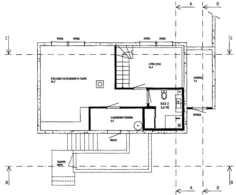
KJELLERPLAN
