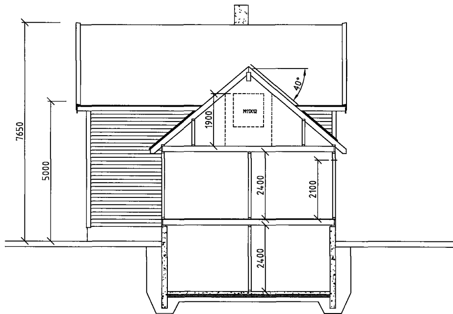
SNITT A-A
