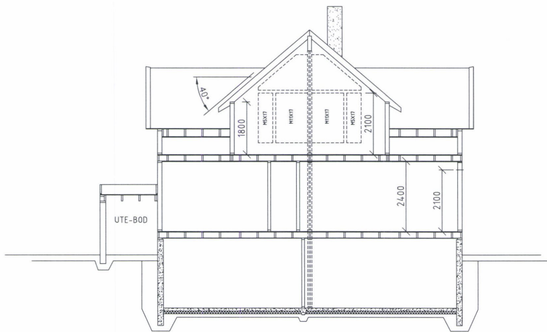
SNITT C-C
