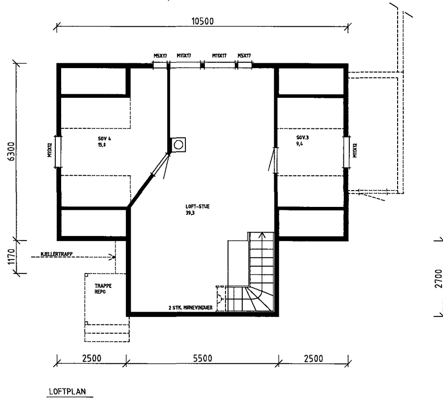
LOFTPLAN
