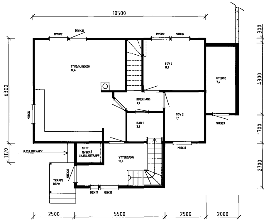
HOVEDPLAN
