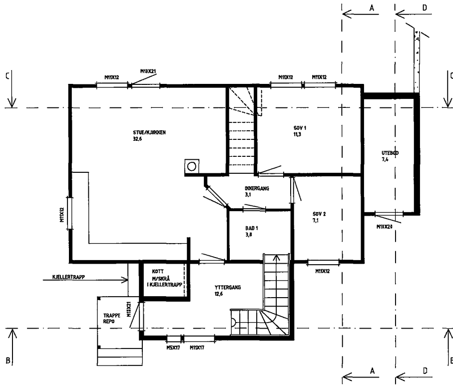
HOVEDPLAN
