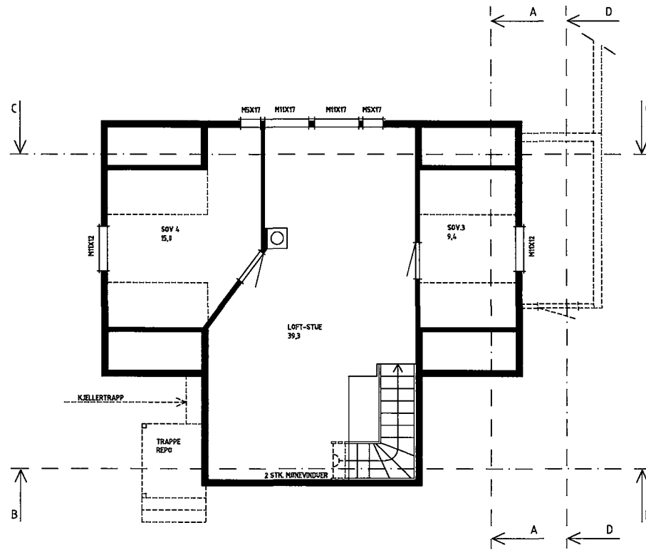
LOFTPLAN
