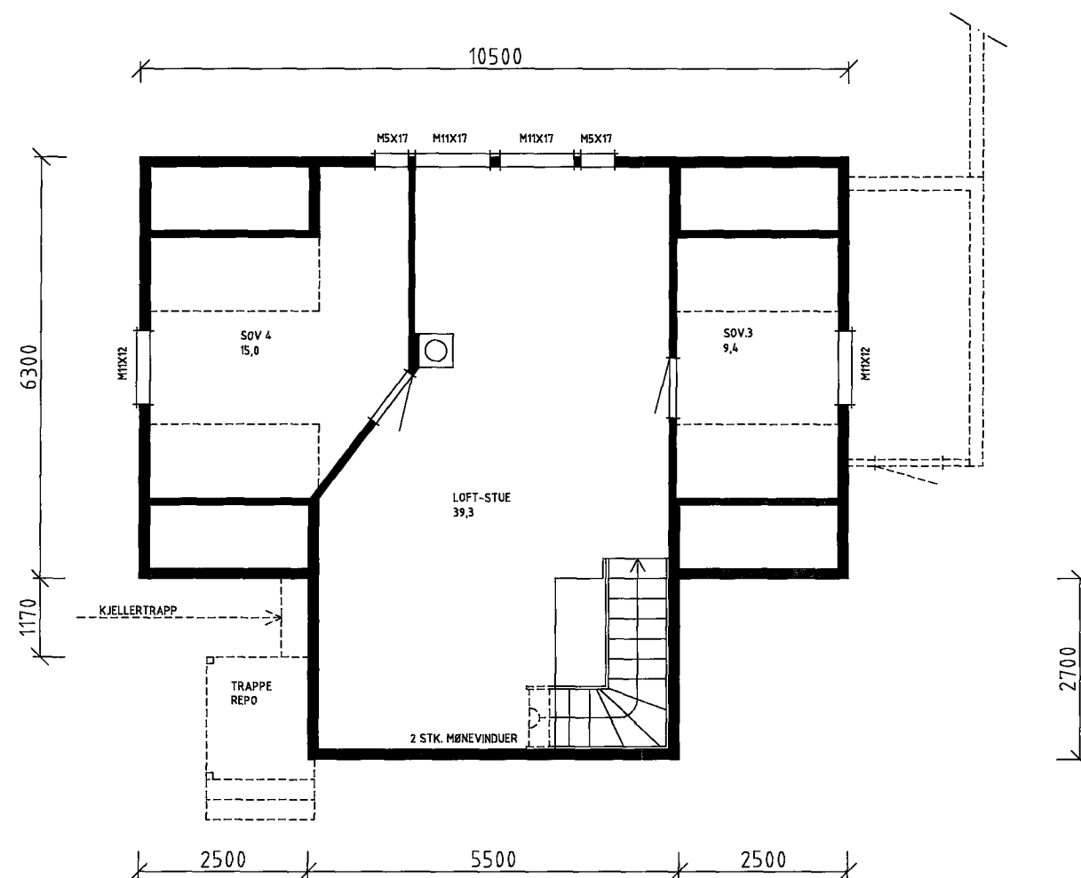
LOFTPLAN
