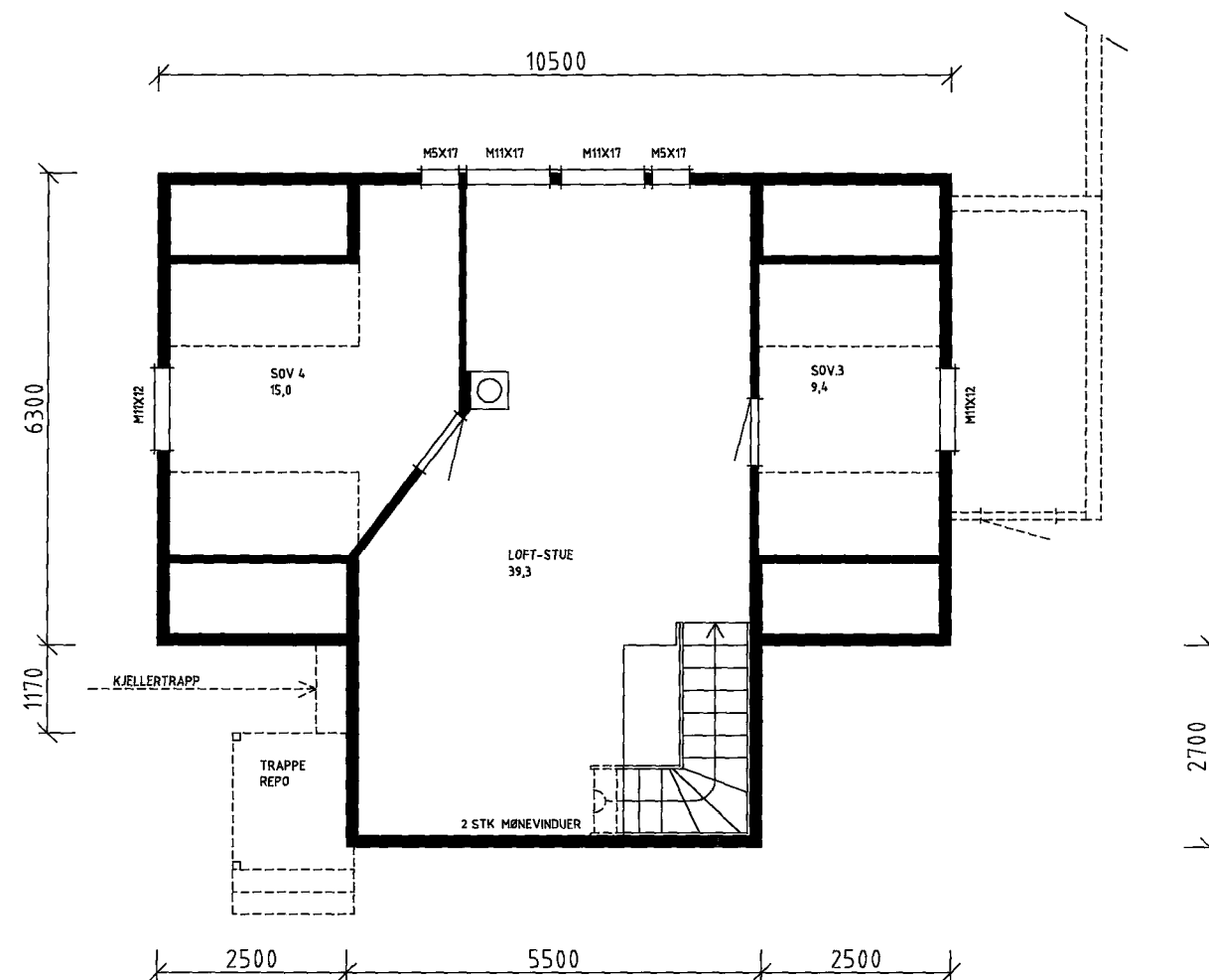
LOFTPLAN
