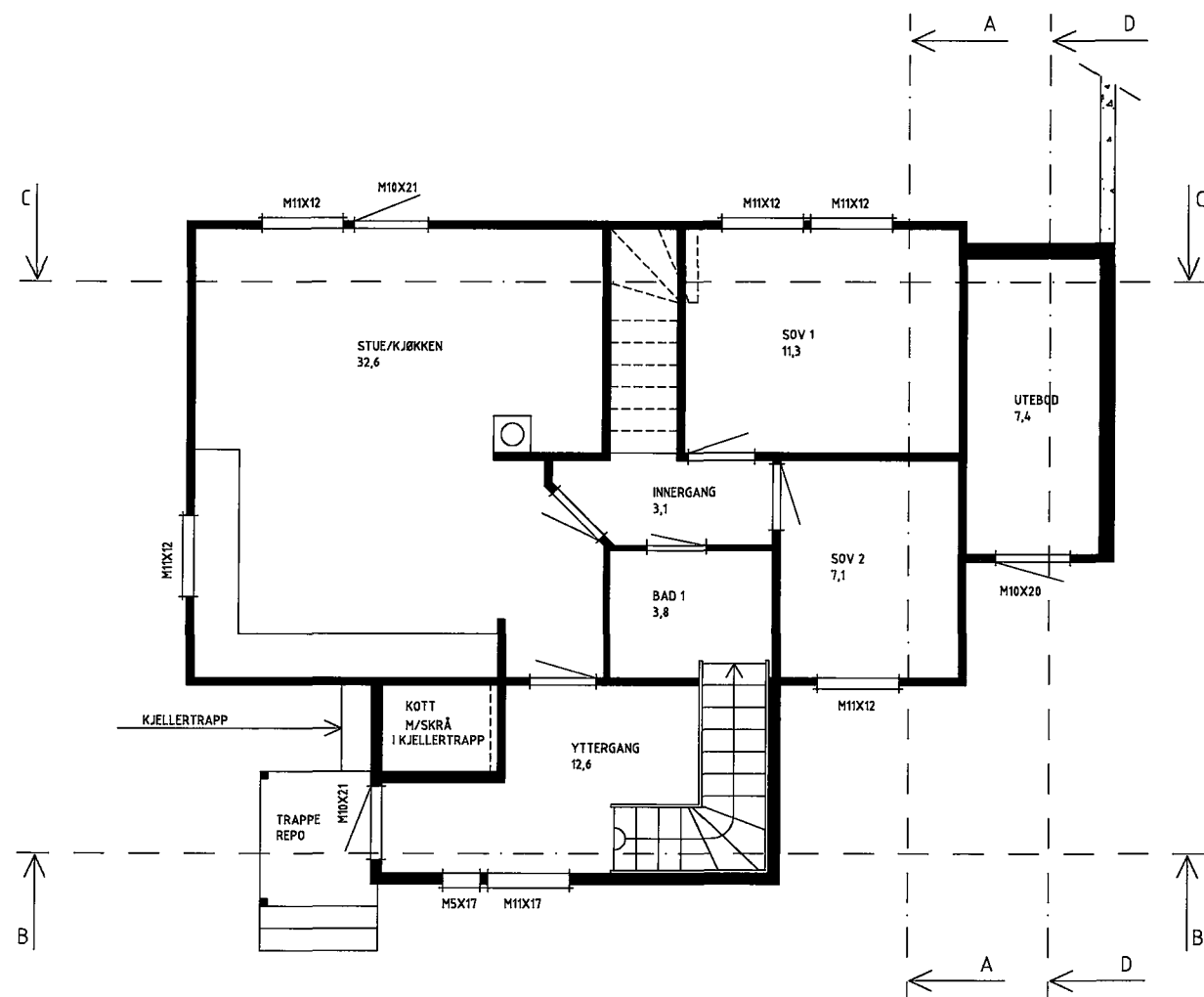
HOVEDPLAN
