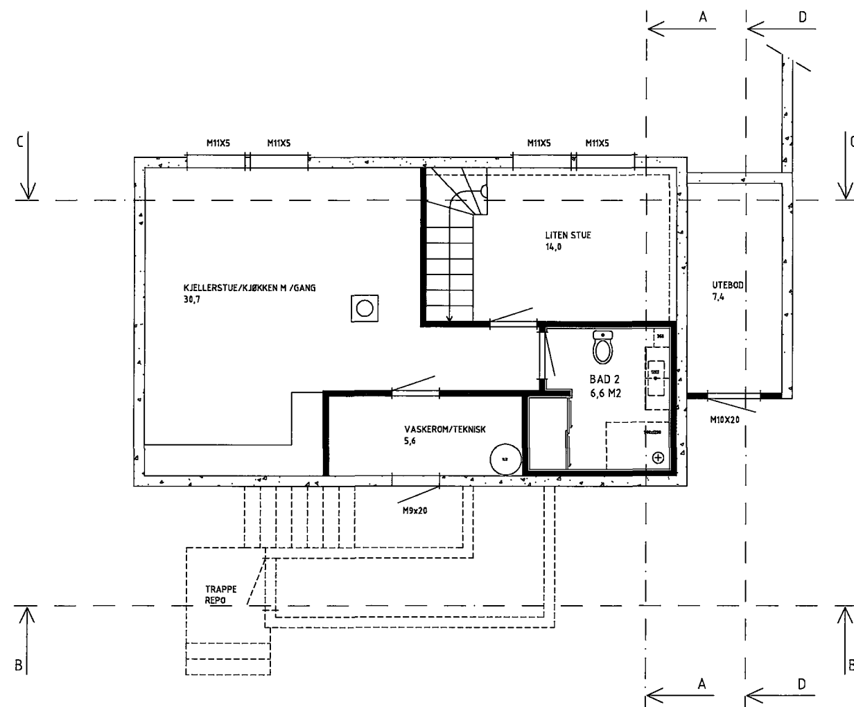
KJELLERPLAN
