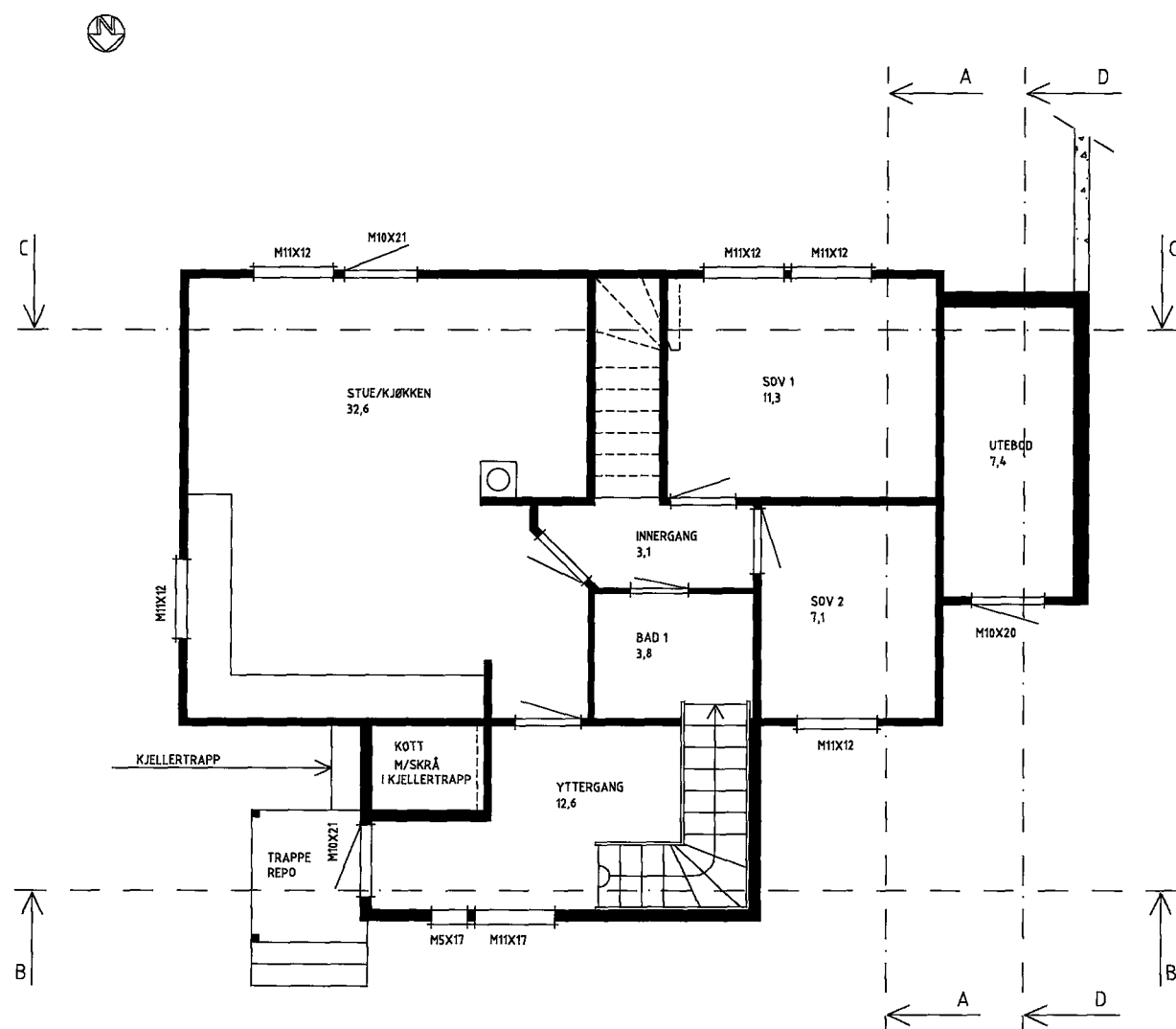
HOVEDPLAN
