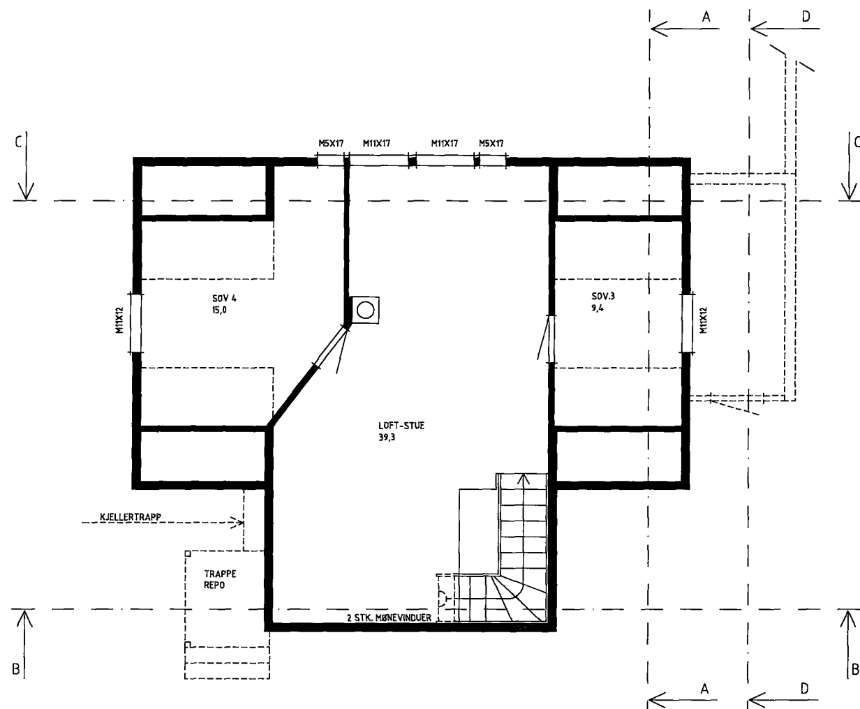
LOFTPLAN
