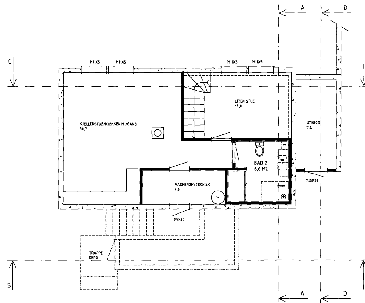
KJELLERPLAN
