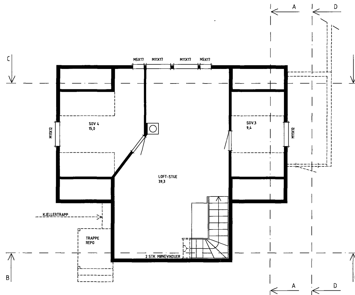
LOFTPLAN
