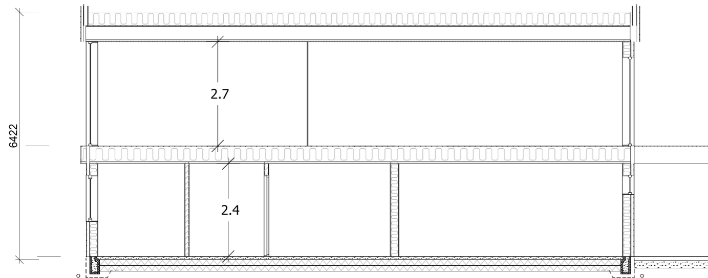
Snitt A:A
