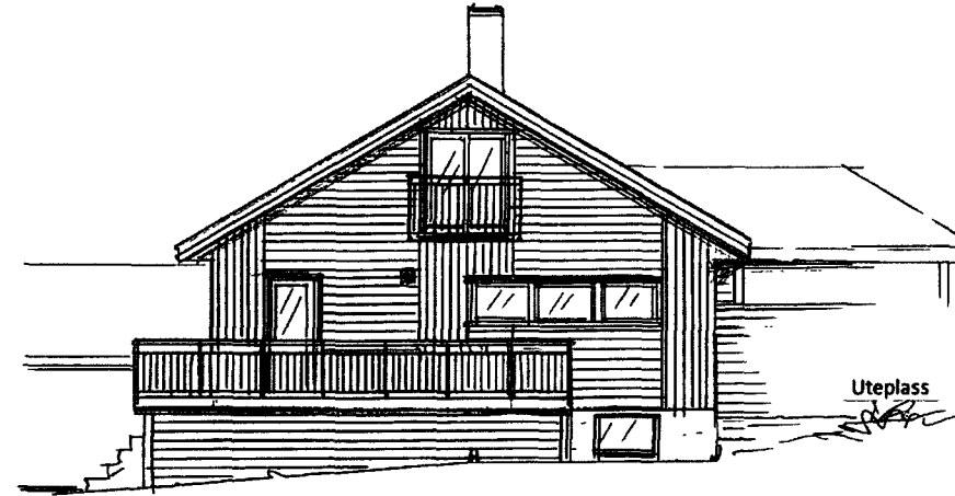
Fasade Vest
