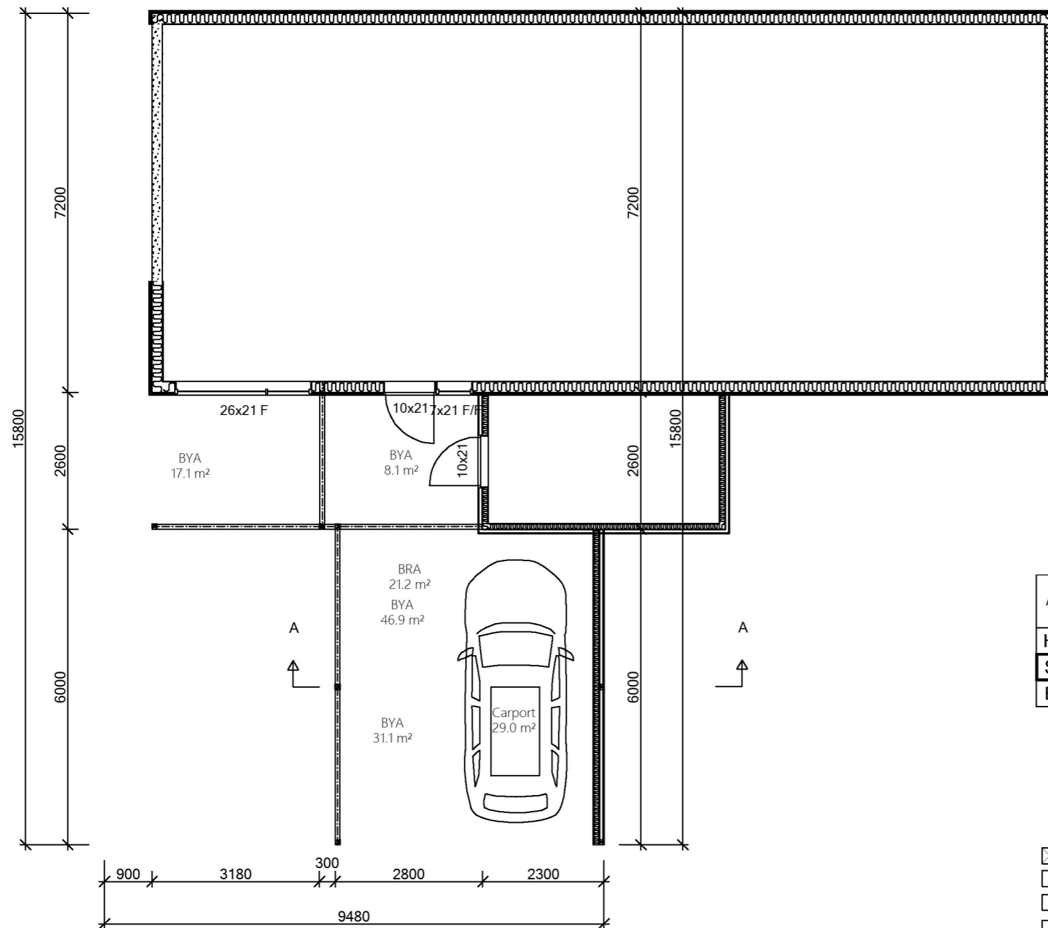
Plan 1. etg.
