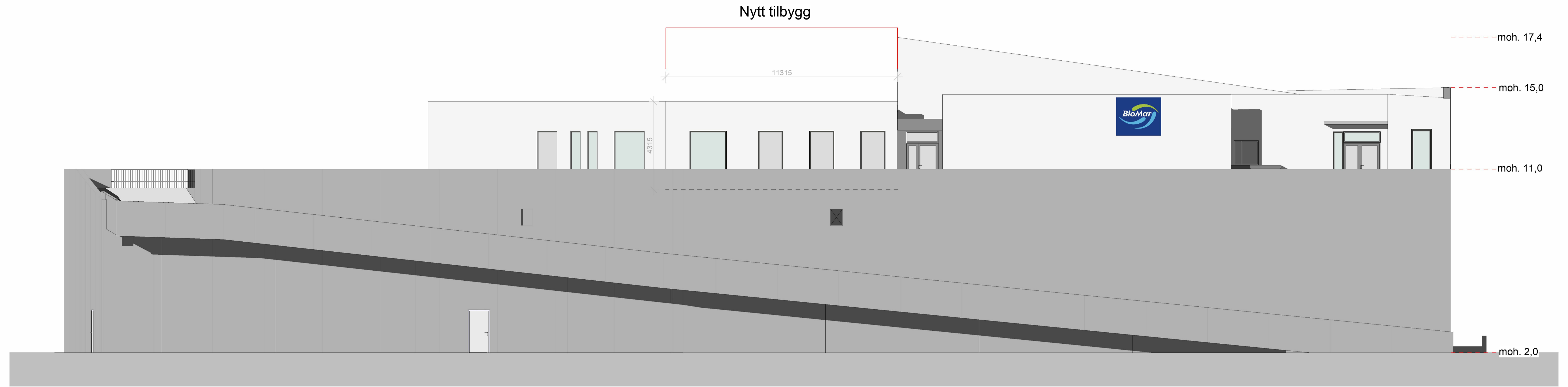
Fasade Tilbygg Nord FA 1 : 100
