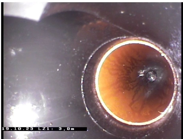
20.10.2023 145146_Endre_Grøft ved gjerde_19102023_073022_004.jpg, 00:00:36, 3.00m Tilkobling. Prefabrikkert grenrør på 12 Kl. / Stakegren i 1B hage
