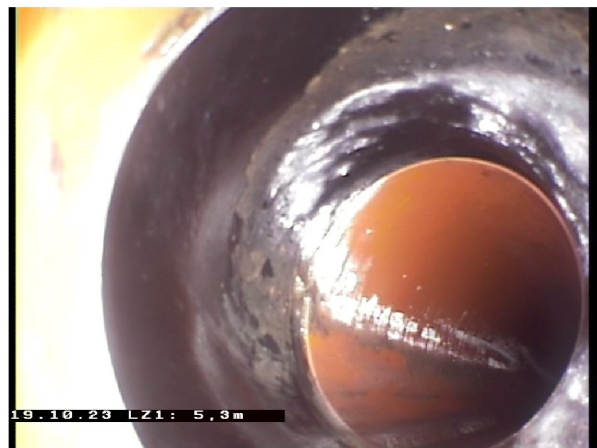
20.10.2023 145146_Endre_Grøft ved gjerde_19102023_073022_005.jpg, 00:00:59, 5.30m Retningsendring. Prefabrikkert kortbend på 3 Kl.
