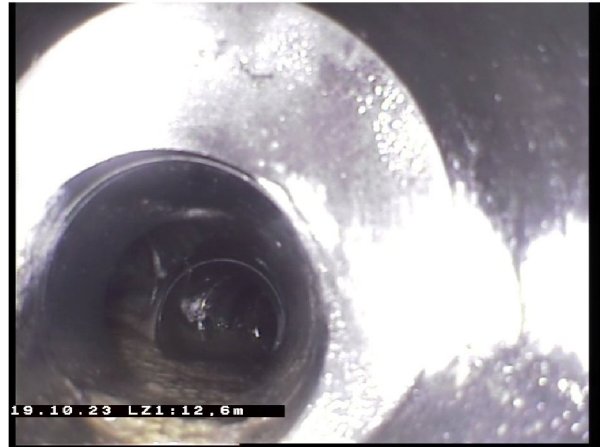
20.10.2023 145146_End_Grøft ved gjerde_19102023_073022_007.jpg, 00:01:55, 12.60m Dimensjonsendring til, S 75 mm
