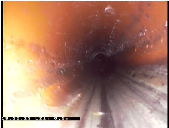
20.10.2023 145146_Endre_Grøft ved gjerde_19102023_073022_002.jpg, 00:00:00, 0.00m Start inspeksjon, 0%
