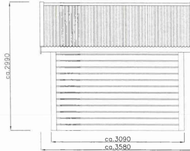
FASADE, SIDEVEGGER.
