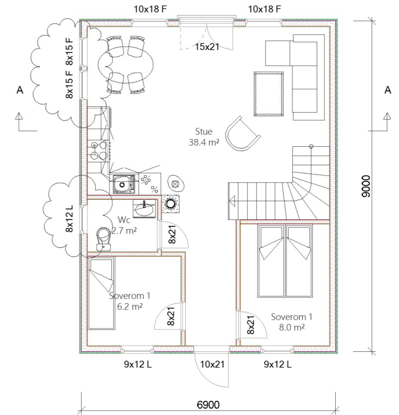
Planløsning hovedetasje
