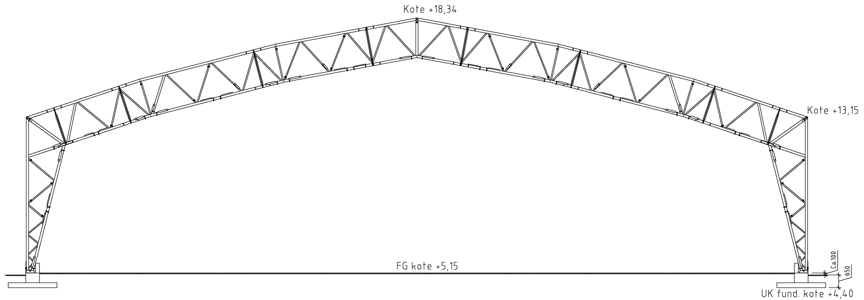
TYPISK SNITT PÅ TVERS AV LAGERHALL
