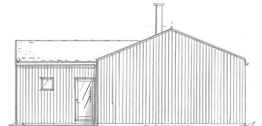
FASADE VEST
