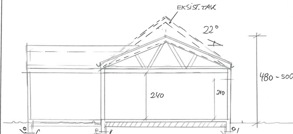
SNITT
