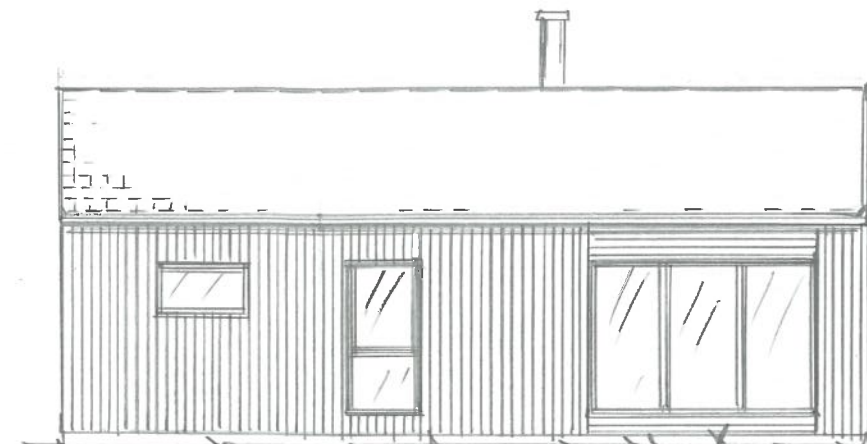
FASADE SØR
