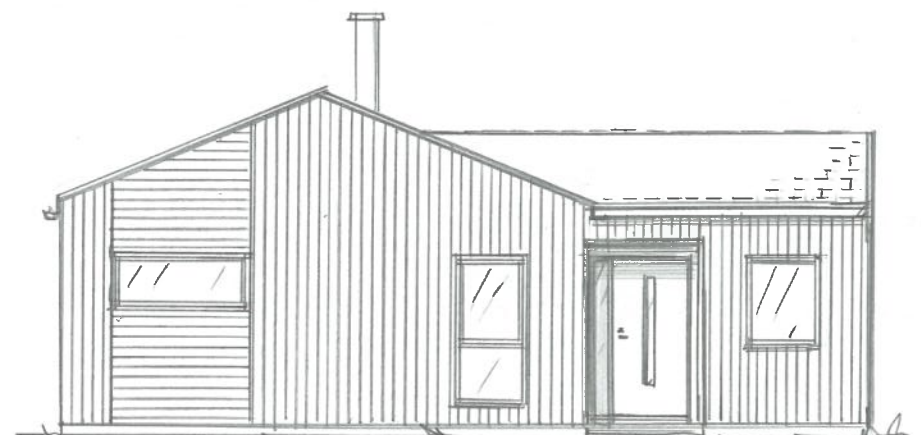
FASADE ØST
