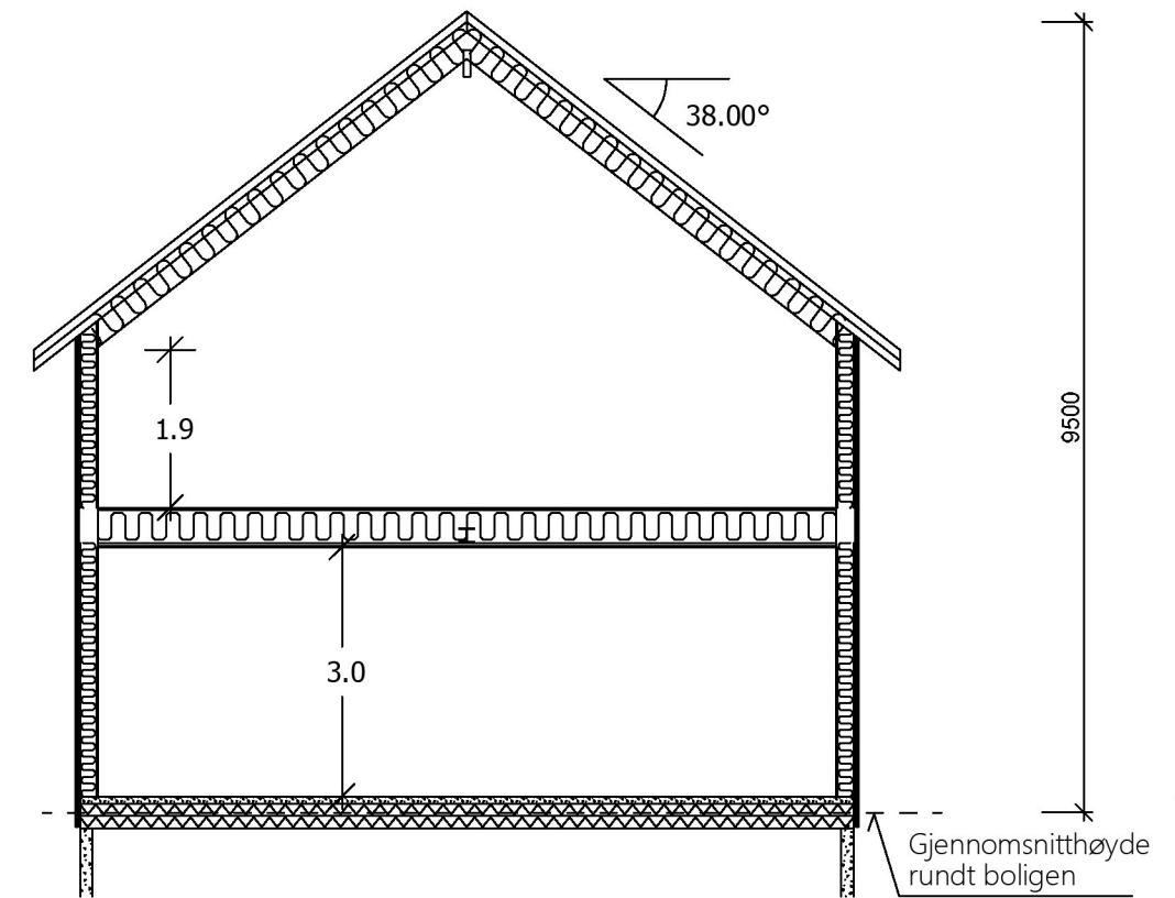
Snitt A:A
